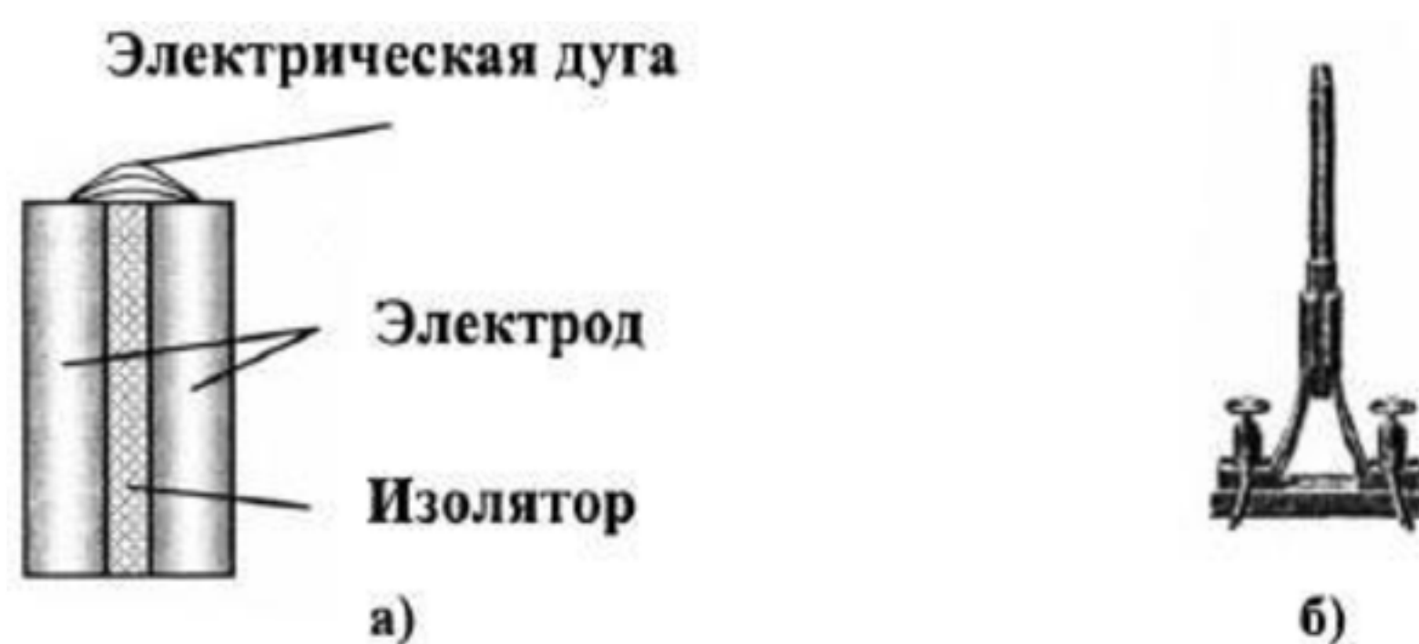
Рис. 4. Свеча Яблочкова
