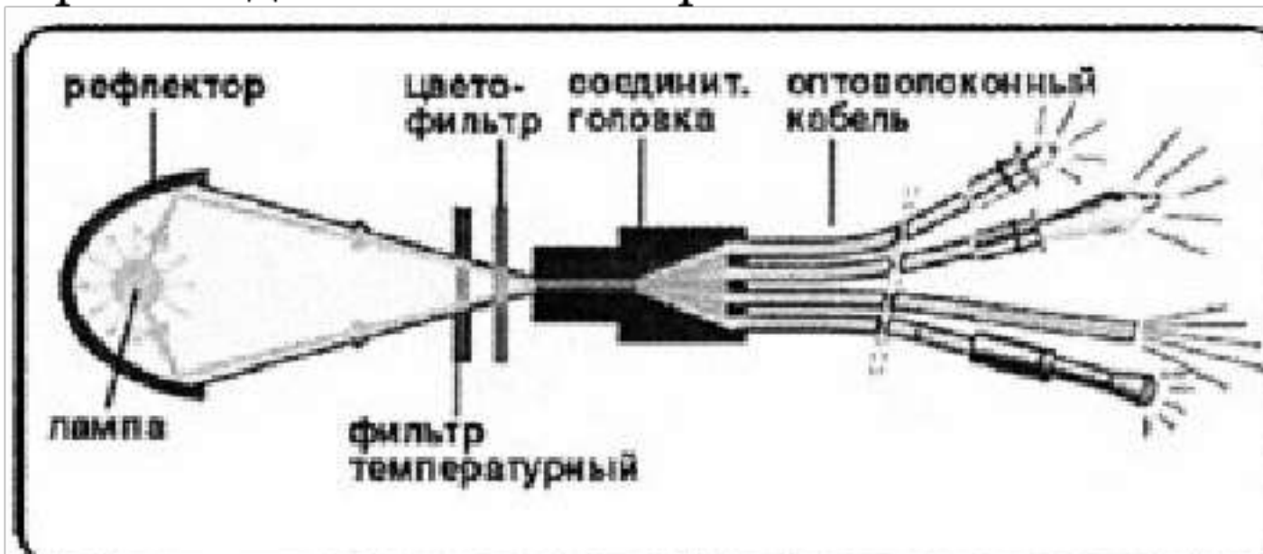
б) схема светильника
