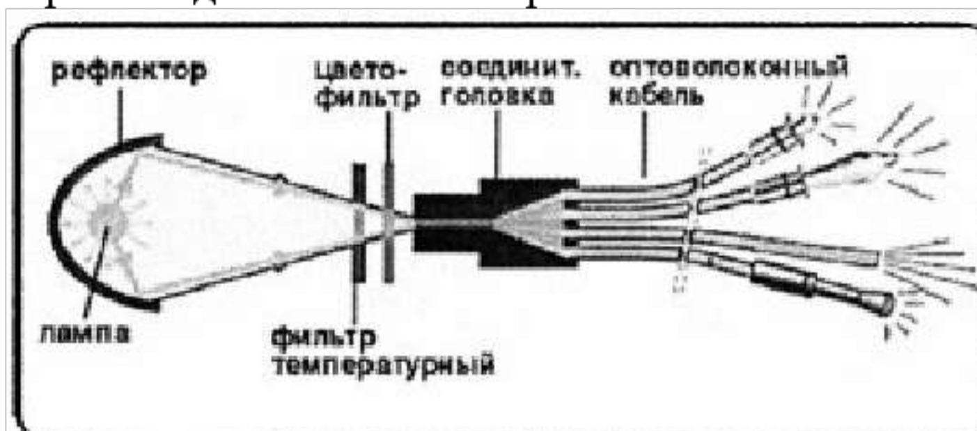
б) схема светильника
