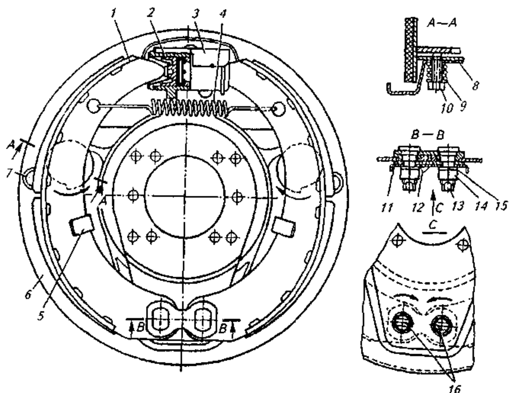
Рис. 3. Тормозной механизм автомобиля ГАЗ-53-12: 1 — тормозная колодка; 2—колесный цилиндр; 3 — экран колесного цилиндра; 4—возвратная пружина колодок; 5—направляющая скоба колодок; 6— тормозной щит; 7—смотровой люк; 8—регулирующий эксцентрик; 9— шайба; 10— болт регулирующего эксцентрика; 11 пластина опорных пальцев; 12 — эксцентрики опорных пальцев; 13 — опорный палец тормозной колодки; 14— гайка; 15— пружинная шайба; 16—метки
