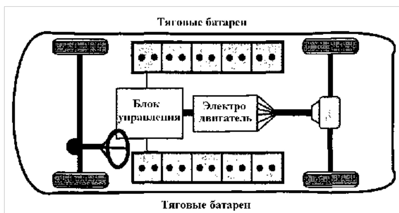
Рис. 1. Компоновочная схема электромотобилия
