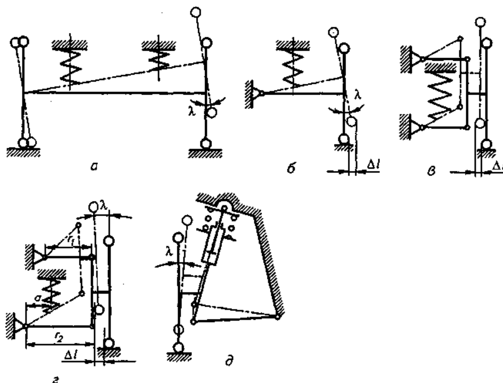
независимая рычажно-телескопическая
