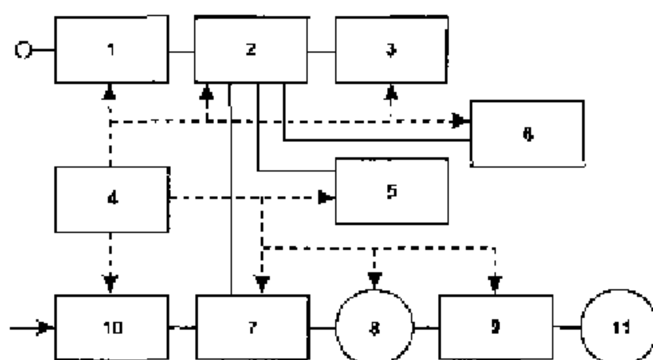
Рис. 2. Блок-схема современного электромотобилия
