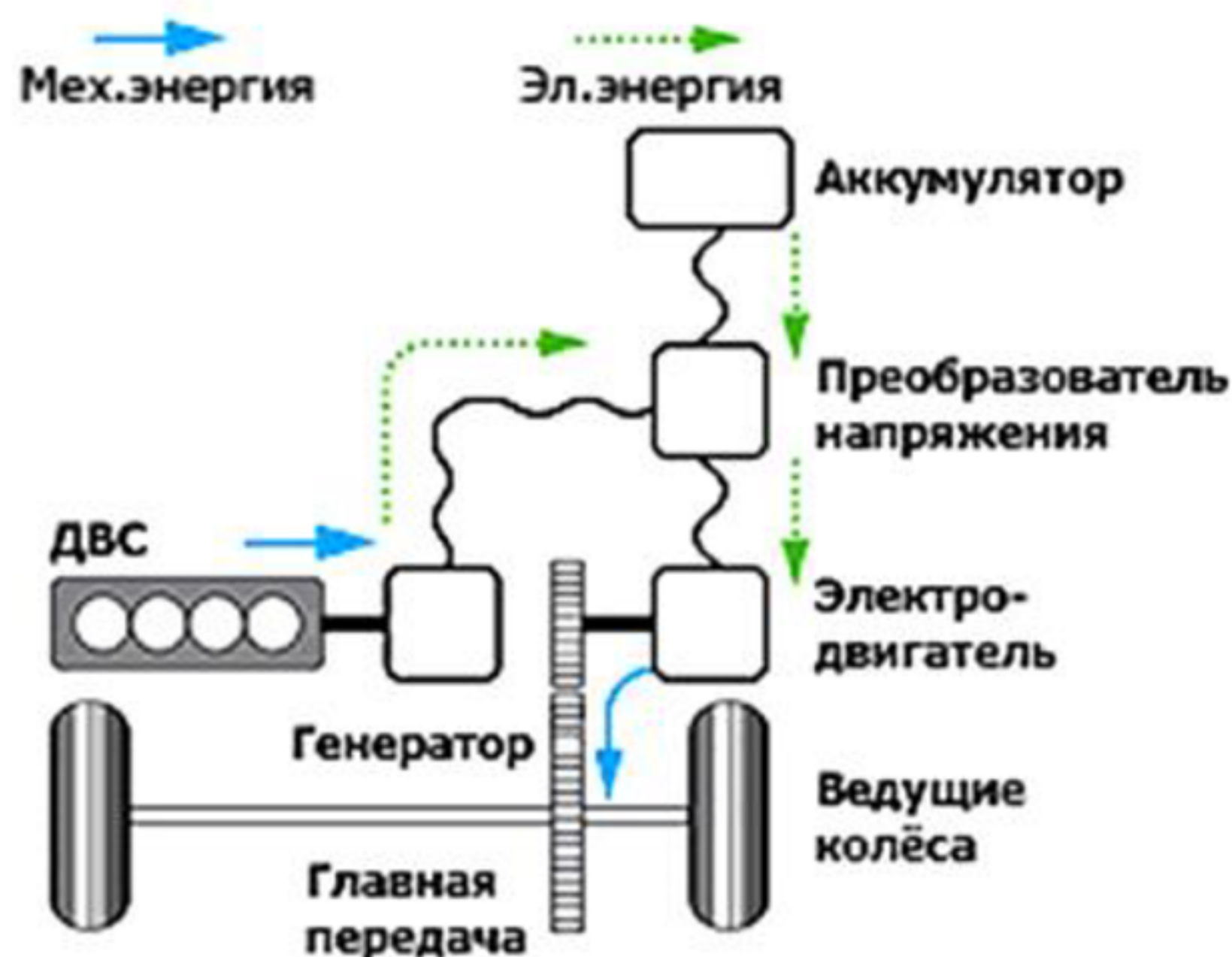
Рис. 3. Принципиальная схема гибридной последовательной силовой установки.
