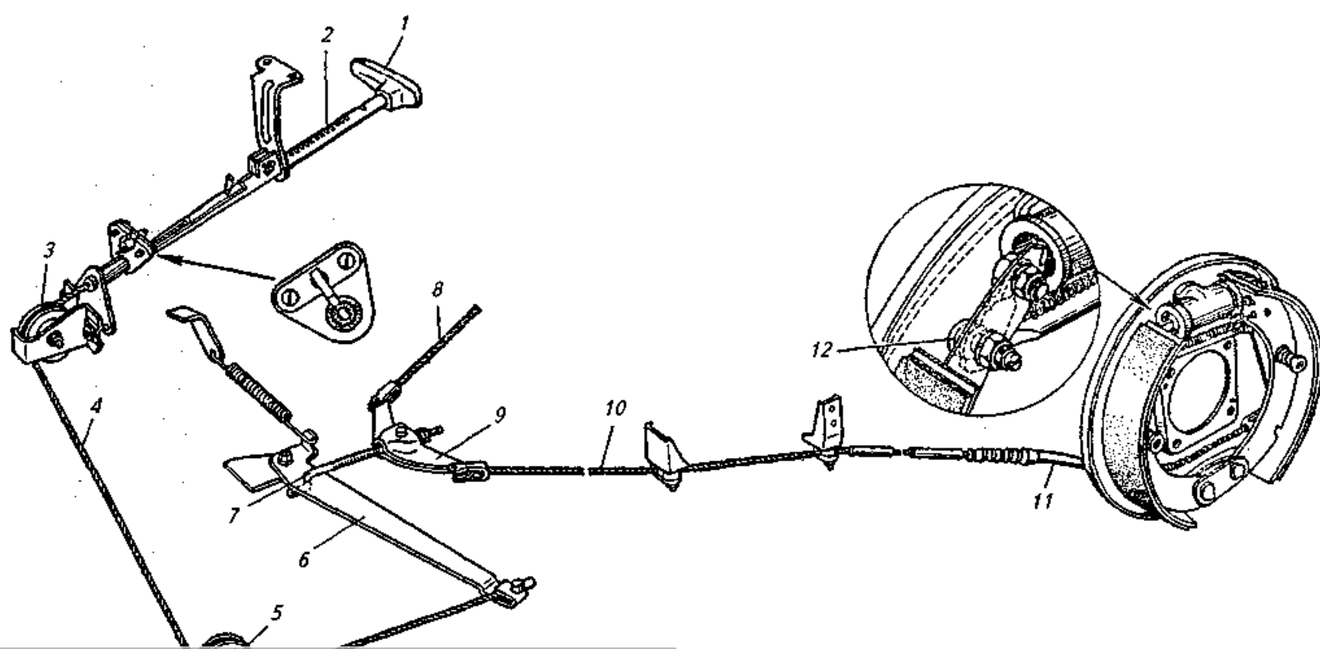
Рис. 25. Стояночный тормоз действующий на задние колеса: 1 — рукоятка; 2 — рычаг; 3, 5 — ролики троса; 4 — передний трос; 6 — промежуточный рычаг; 7 — стержень; 8, 10 — ролики троса; 9 — уравниватель тормоза; 11 — трубка; 12 — эксцентриковая ось разжимного рычага
