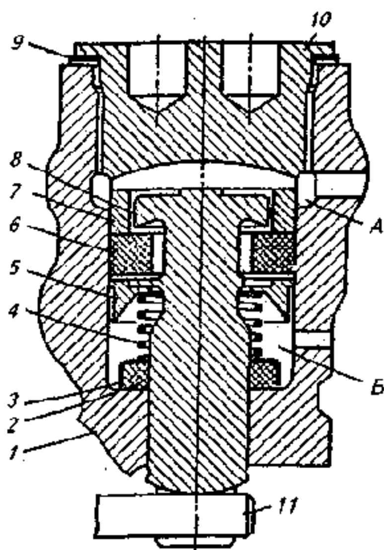
Рис. 21. Регулятор давления автомобиля ВАЗ-2121: А, Б- полости регулятора; 1 — корпус; 2—уплотнительное кольцо; 3— обойма; 4— пружина; 5—тарелка; 6 — резиновый уплотнитель; 7-распорная втулка; 8— поршень; 9—прокладка; 10— пробка; 11 — торсион привода регулятора
