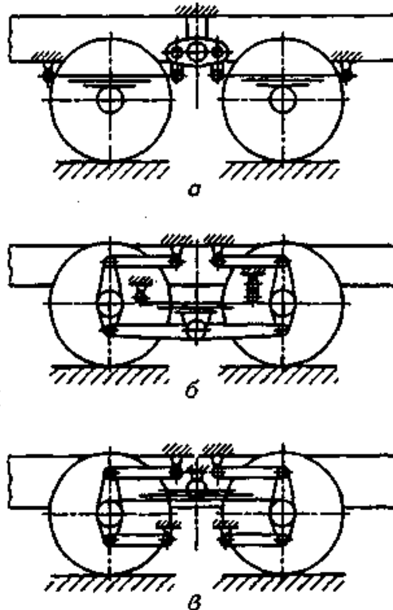
Рис. 14. Схемы четырехрессорная жесткой балансирными
