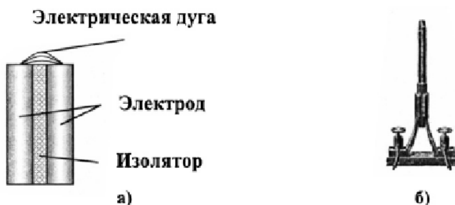
Рис. 4. Свеча Яблочкова
