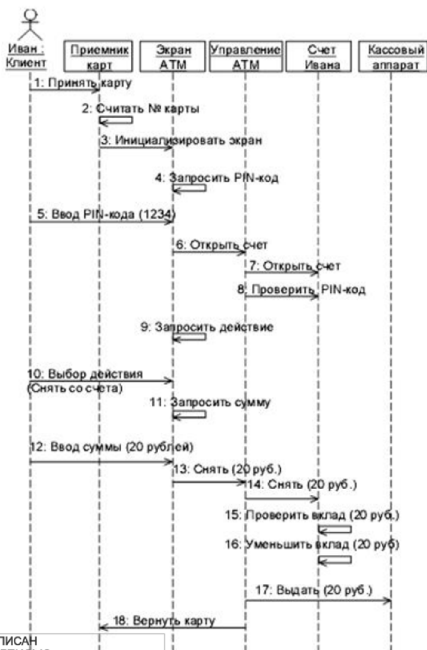
Рисунок 3.7 - Пример диаграммы последовательности
