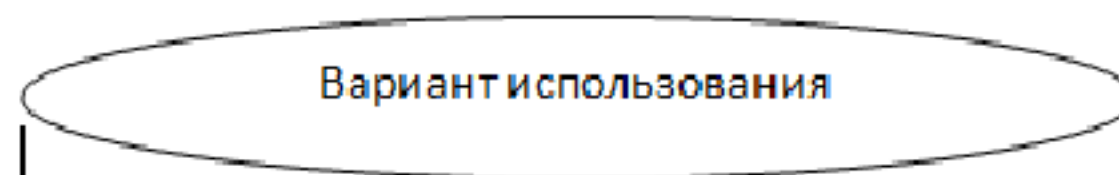
Рисунок 3.2 - Вариант использования
