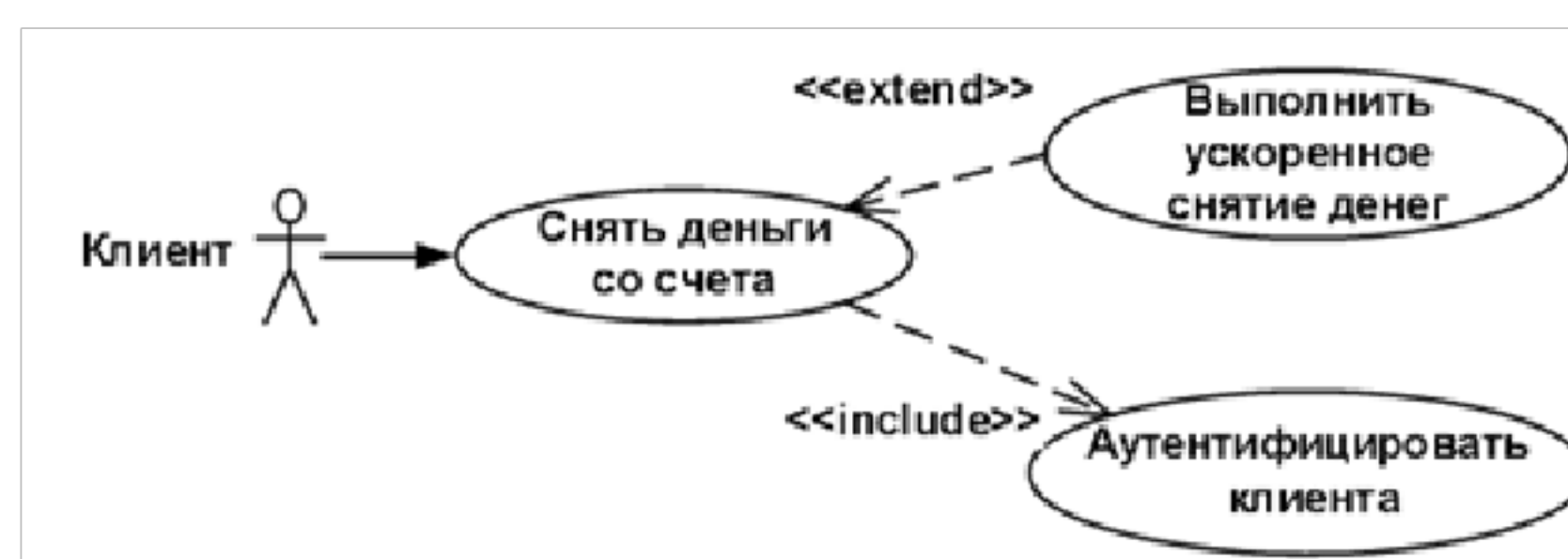
Рисунок 3.5 - Пример связи включения и расширения
