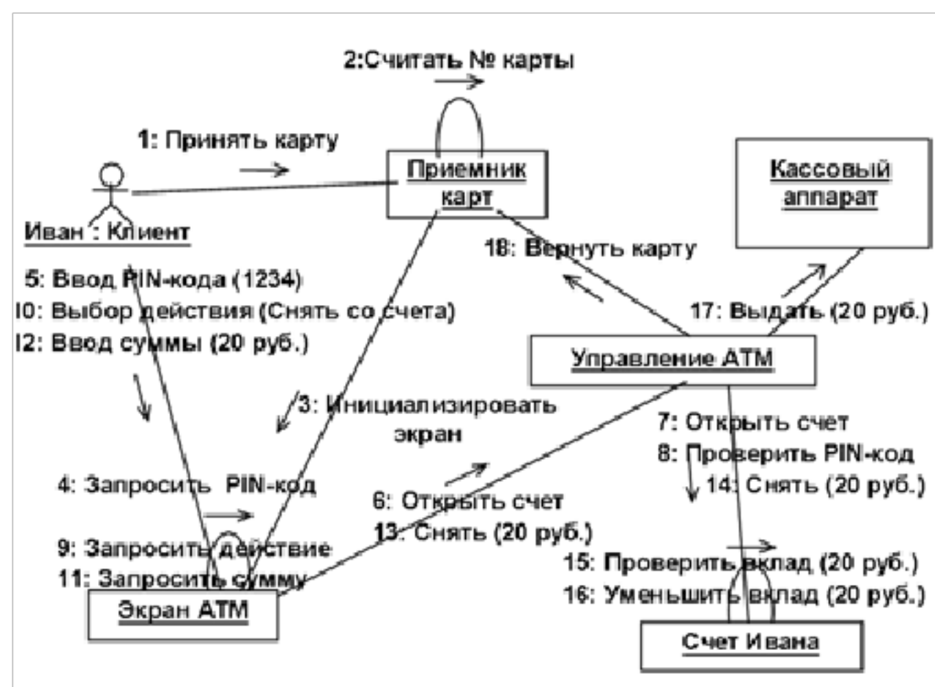
Рисунок 3.8 - Пример диаграммы кооперации
