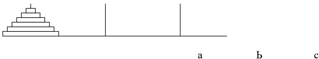
Рис. 4. Ханойская башня
