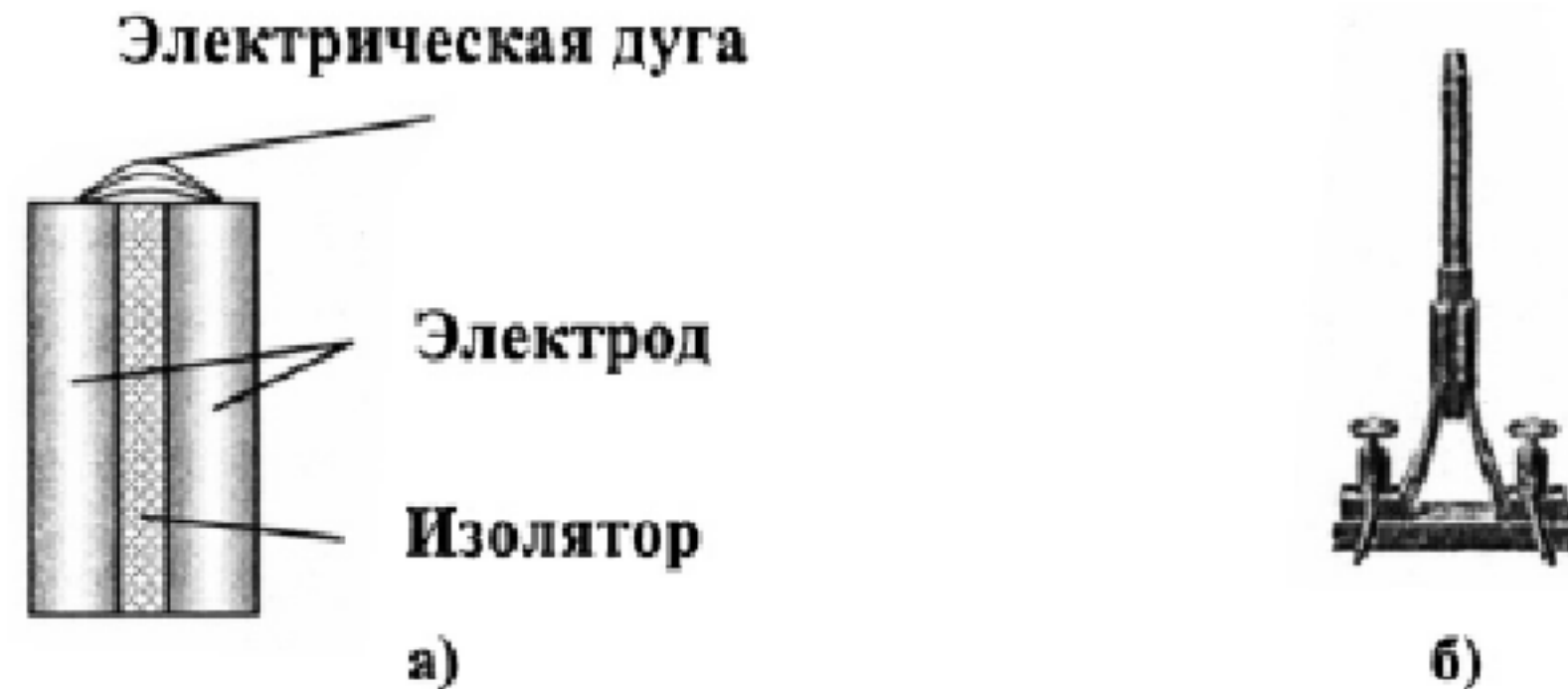
Рис. 4. Свеча Яблочкова
