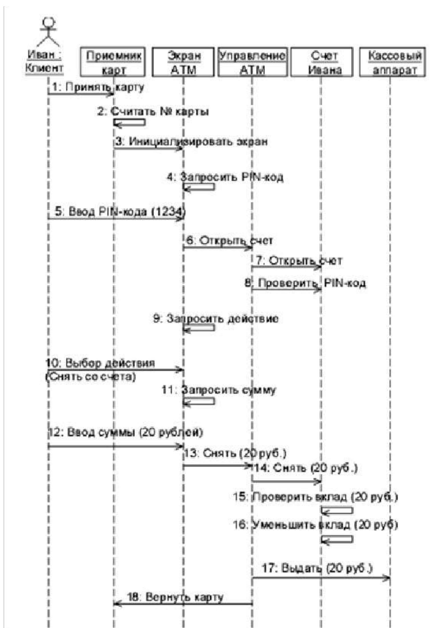
Рисунок 3.7 - Пример диаграммы последовательности
