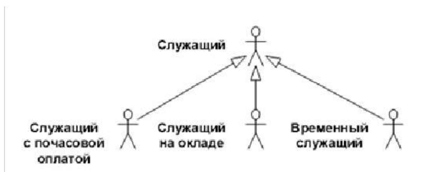
Рисунок 3.6 - Пример связи обобщения
