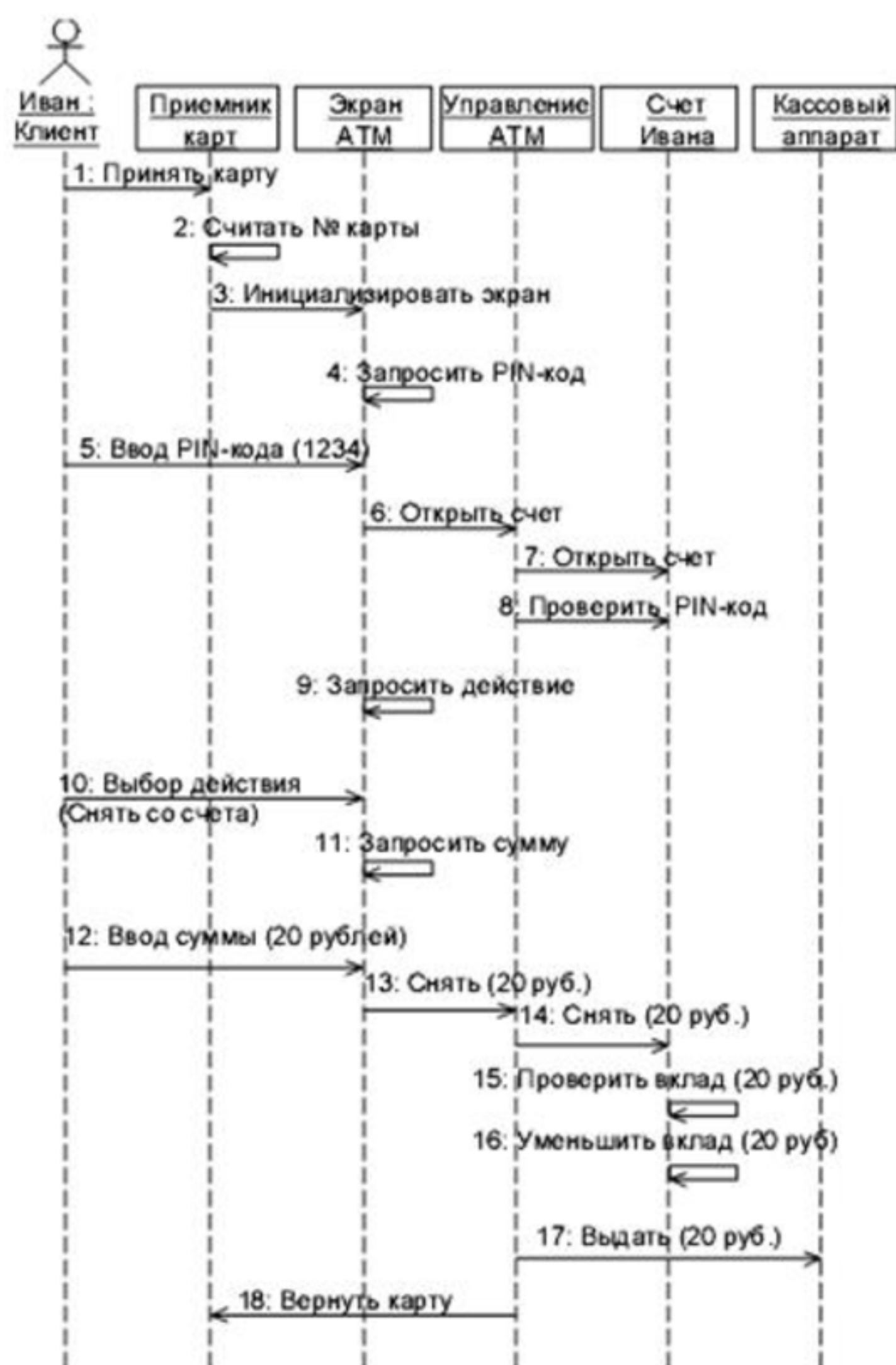
Рисунок 2.7 - Пример диаграммы последовательности
