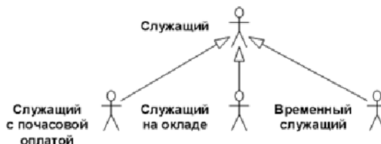
Рисунок 3.6 - Пример связи обобщения
