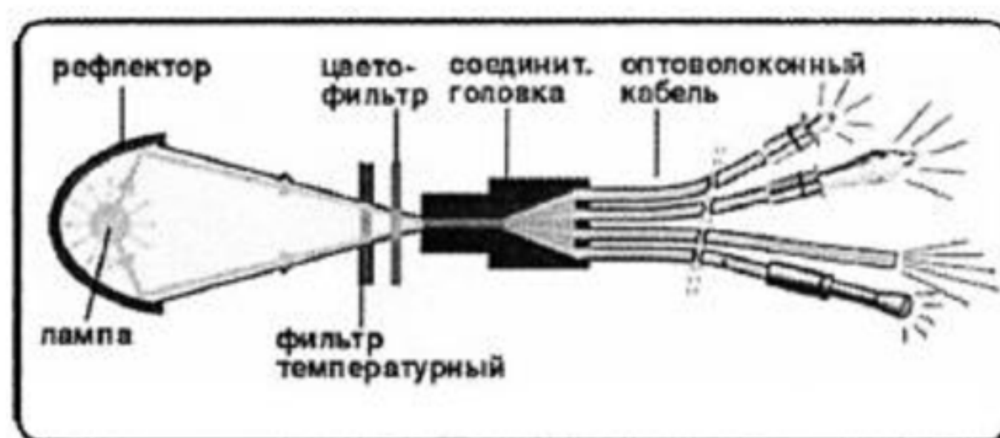
а) схема светильника
