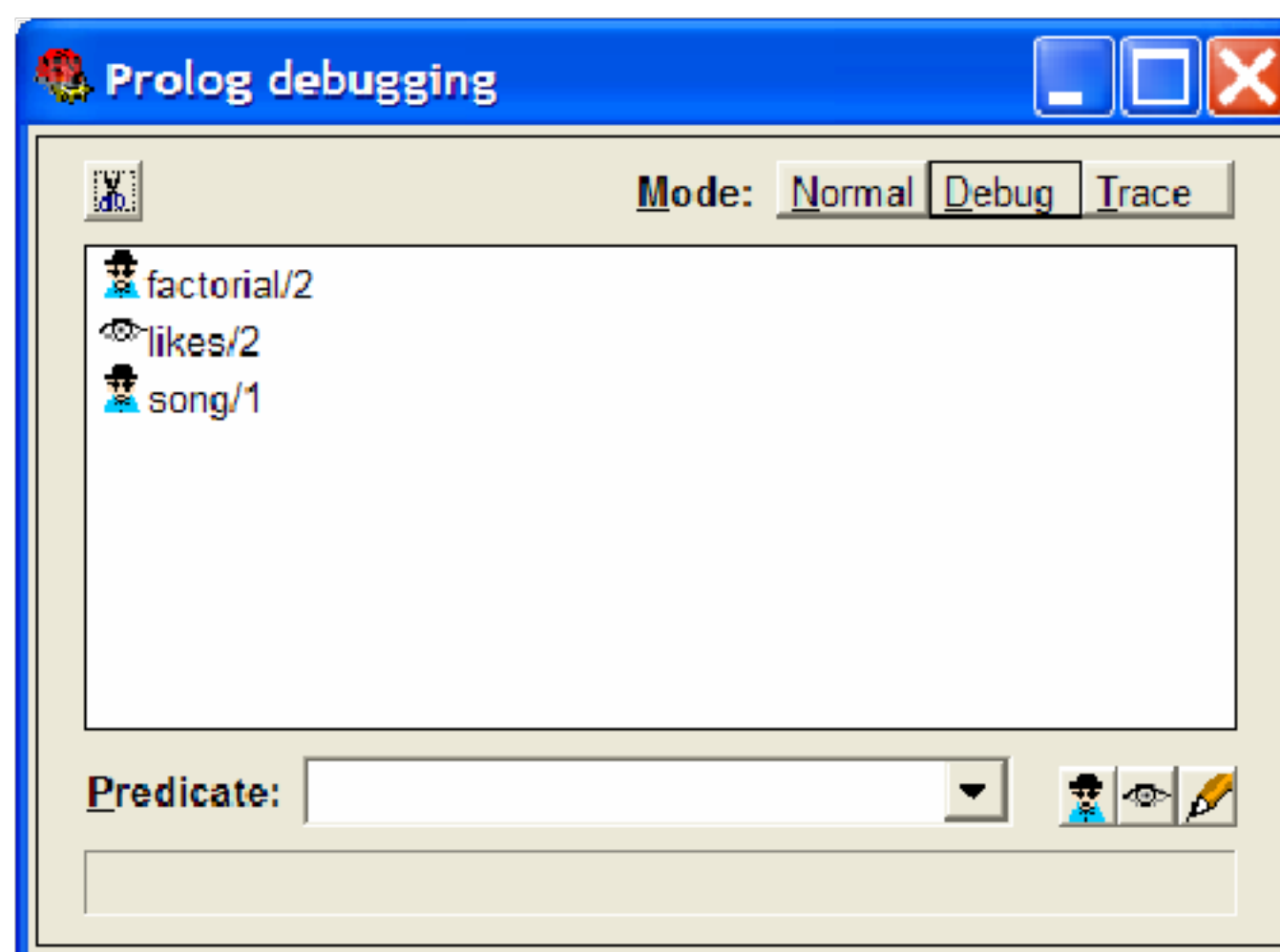
Рисунок 1.5 – Режим трассировки
