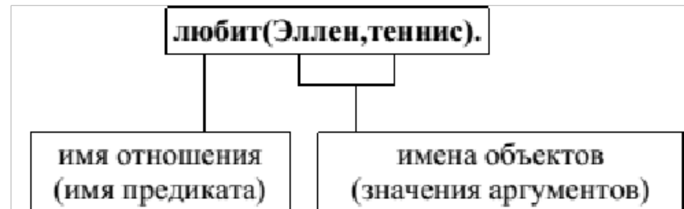
Рисунок 1.2 – Синтаксис Пролог
