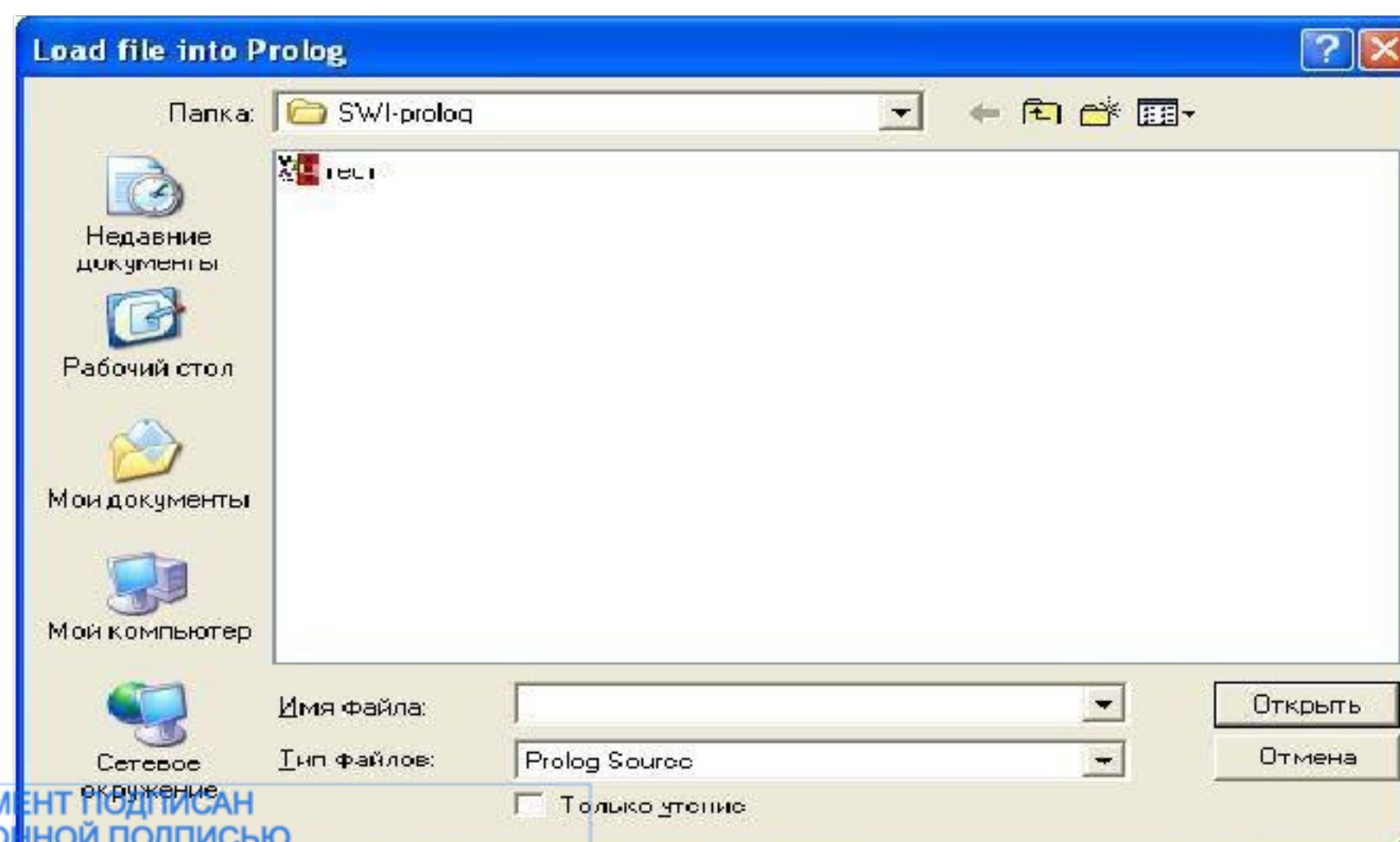
Рисунок 1.3 - Диалоговое окно
