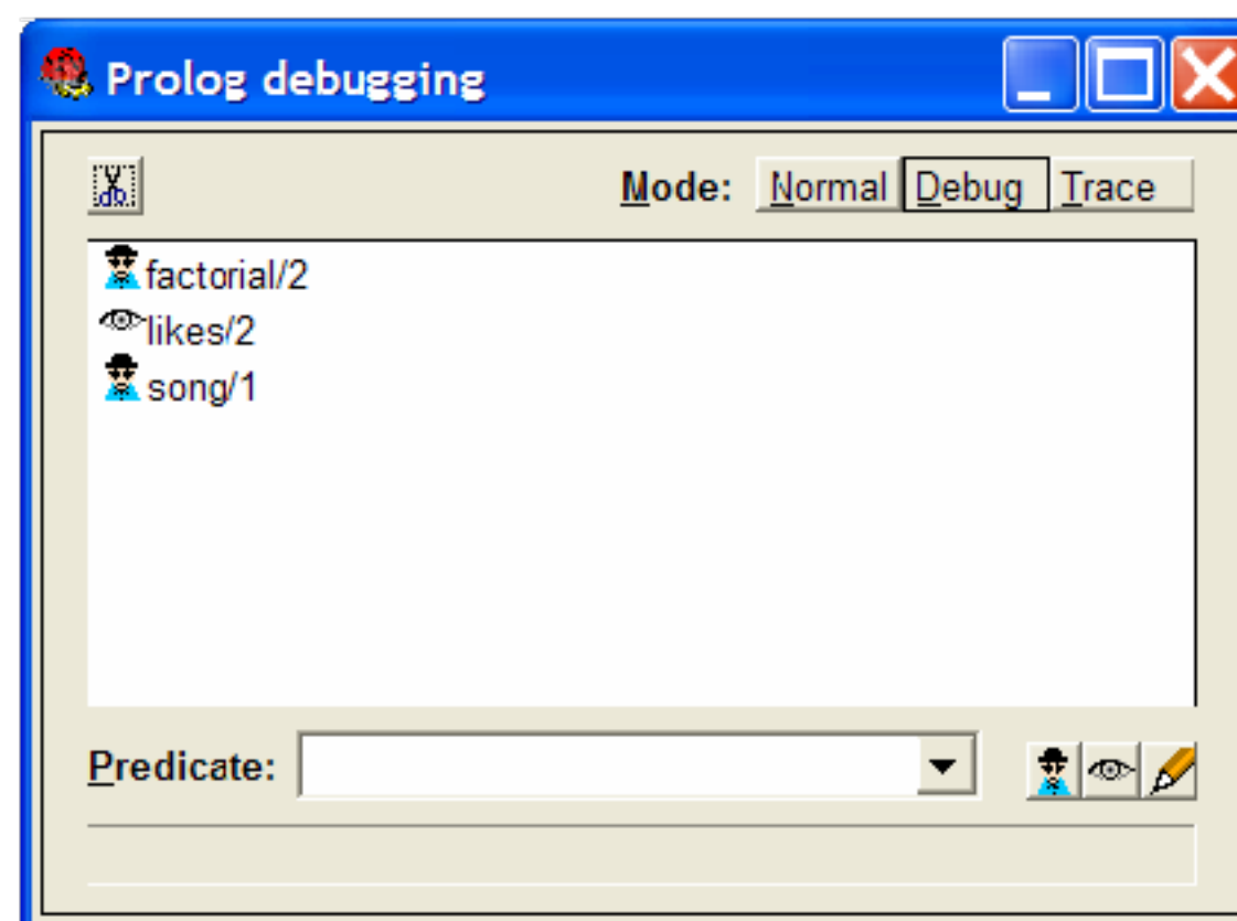
Рисунок 1.5 – Режим трассировки
