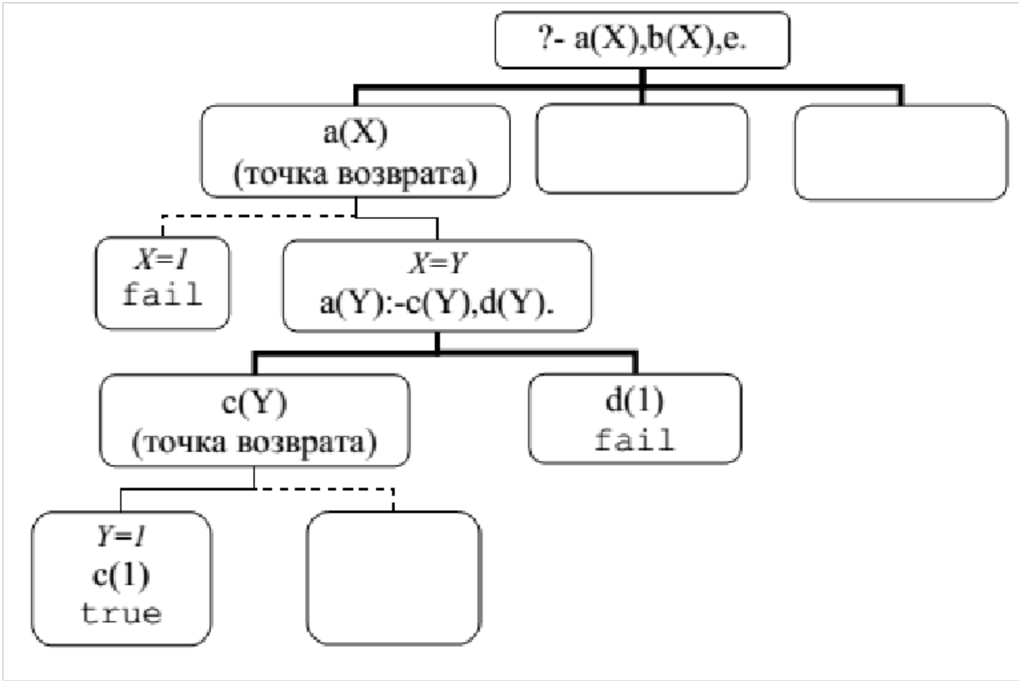
Рисунок 1.7 – Выполнение программы
