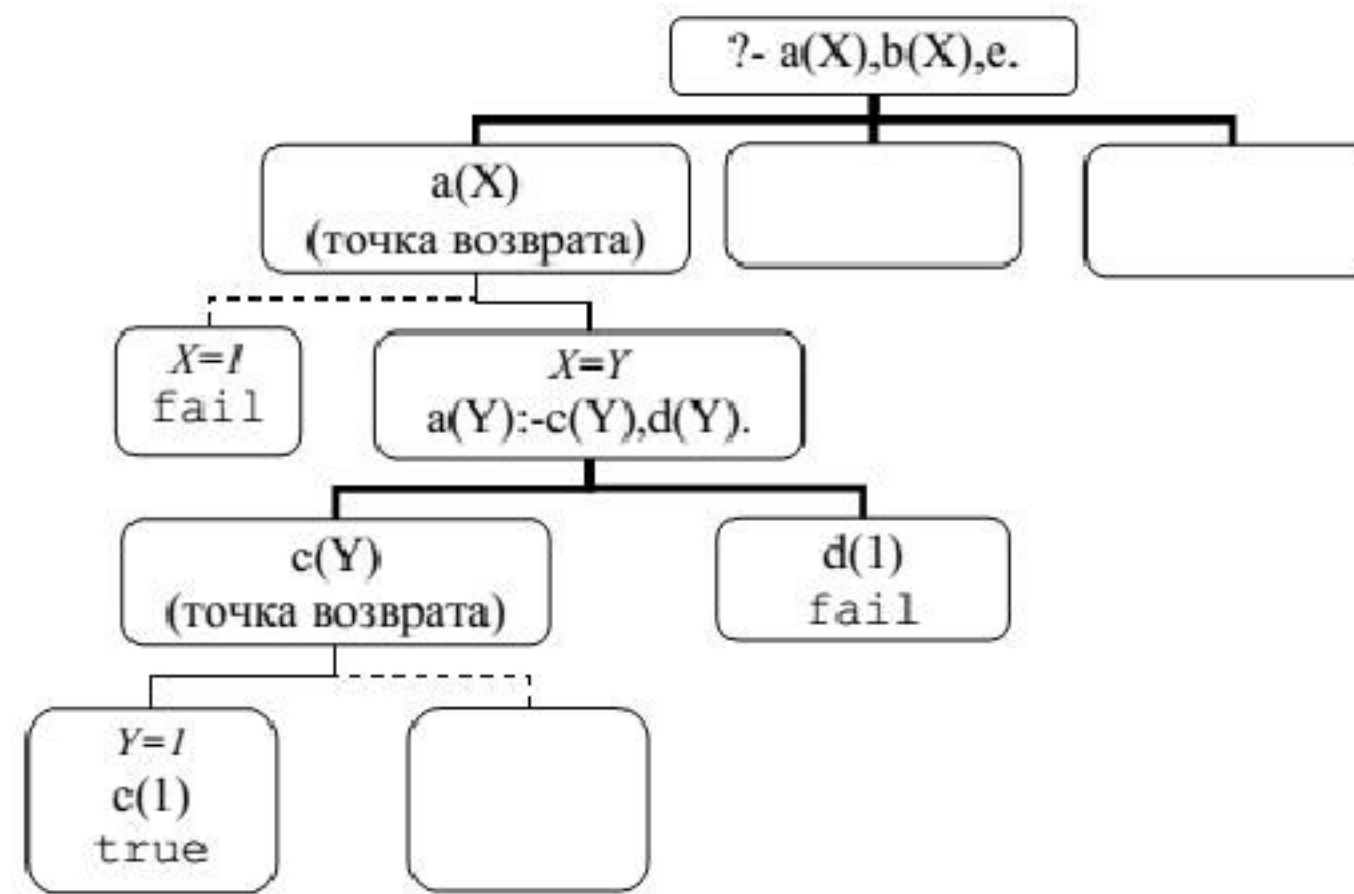
Рисунок 1.7 – Выполнение программы
