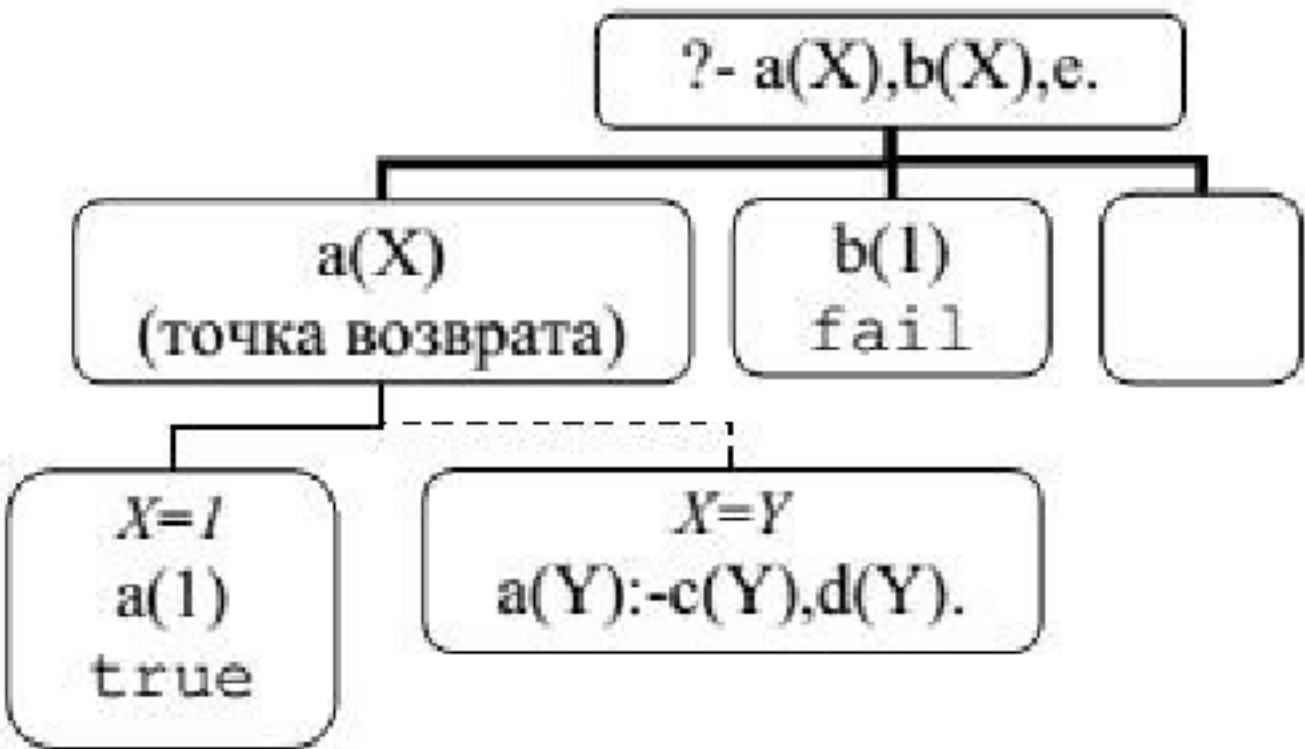
Рисунок 1.6 – Выполнение программы
