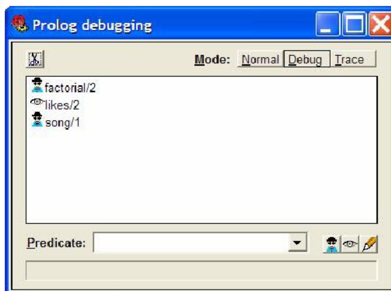
Рисунок 1.5 – Режим трассировки
