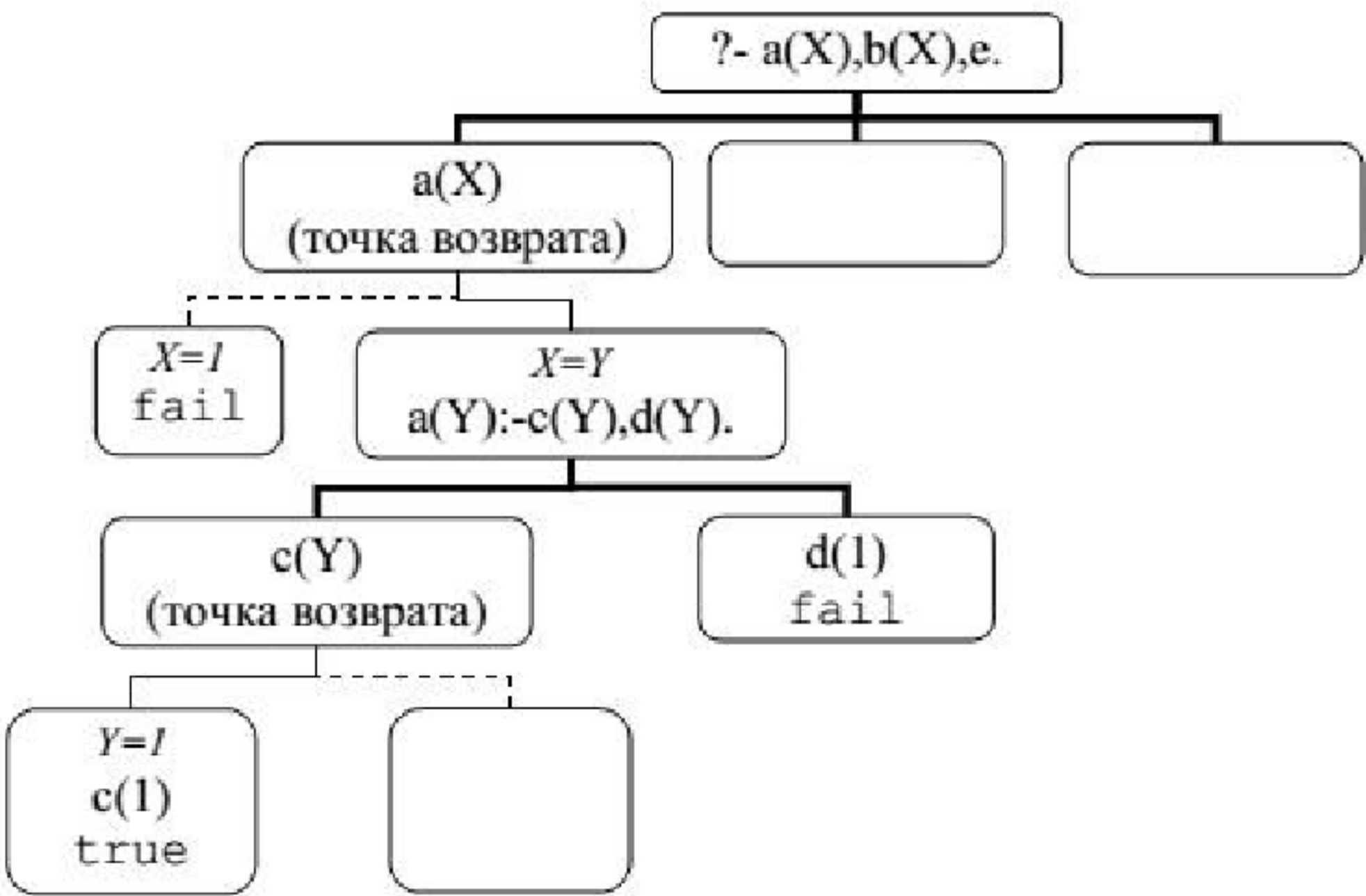
Рисунок 1.7 – Выполнение программы
