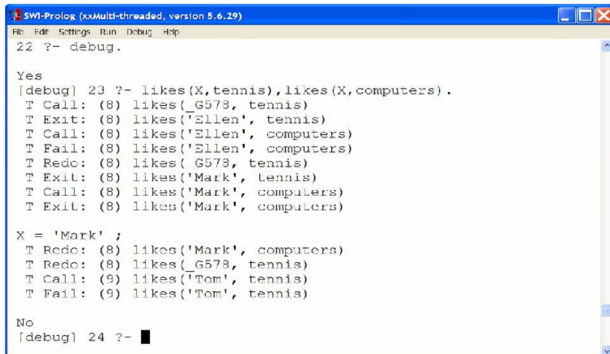
Рисунок 1.7 – Трассировка программы
