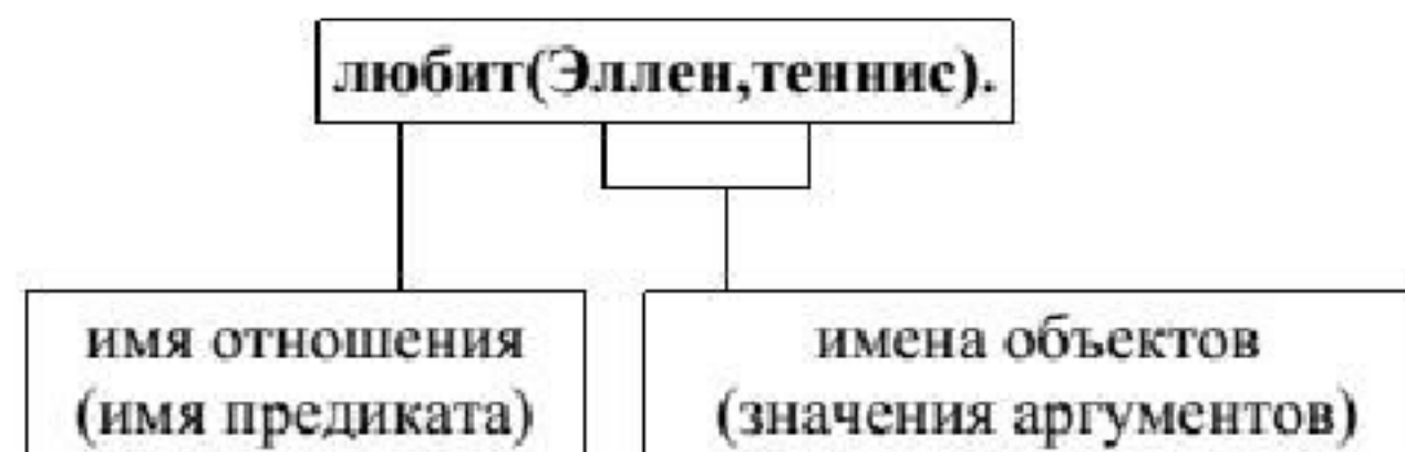
Рисунок 1.2 – Синтаксис Пролог
