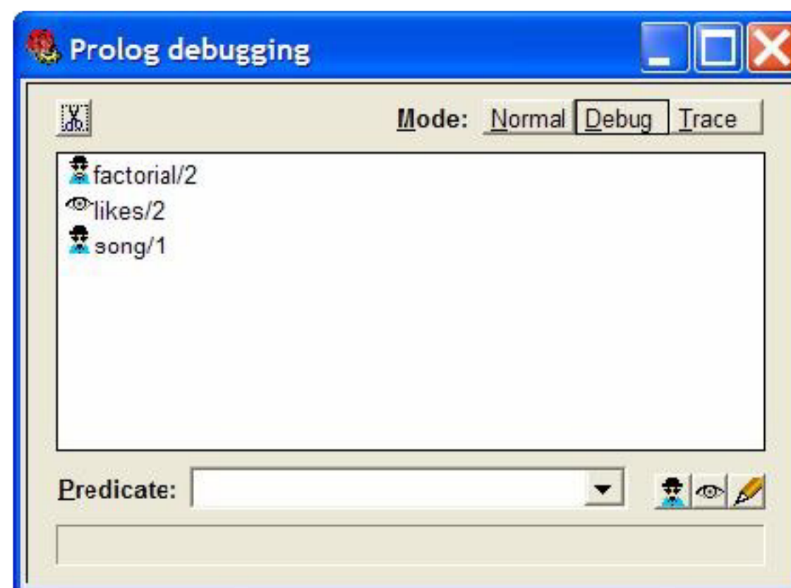
Рисунок 1.5 – Режим трассировки
