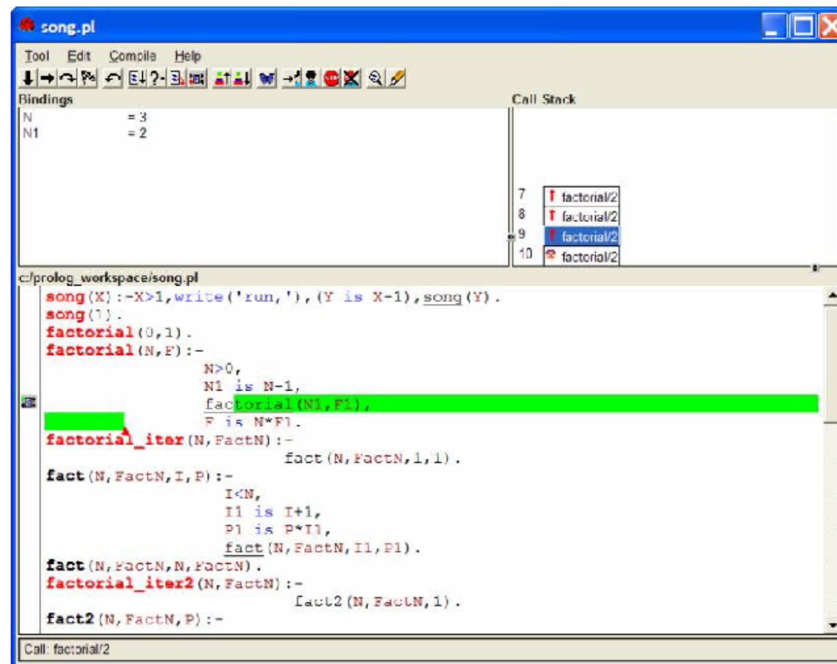
Рисунок 1.8 – Результат трассировки
