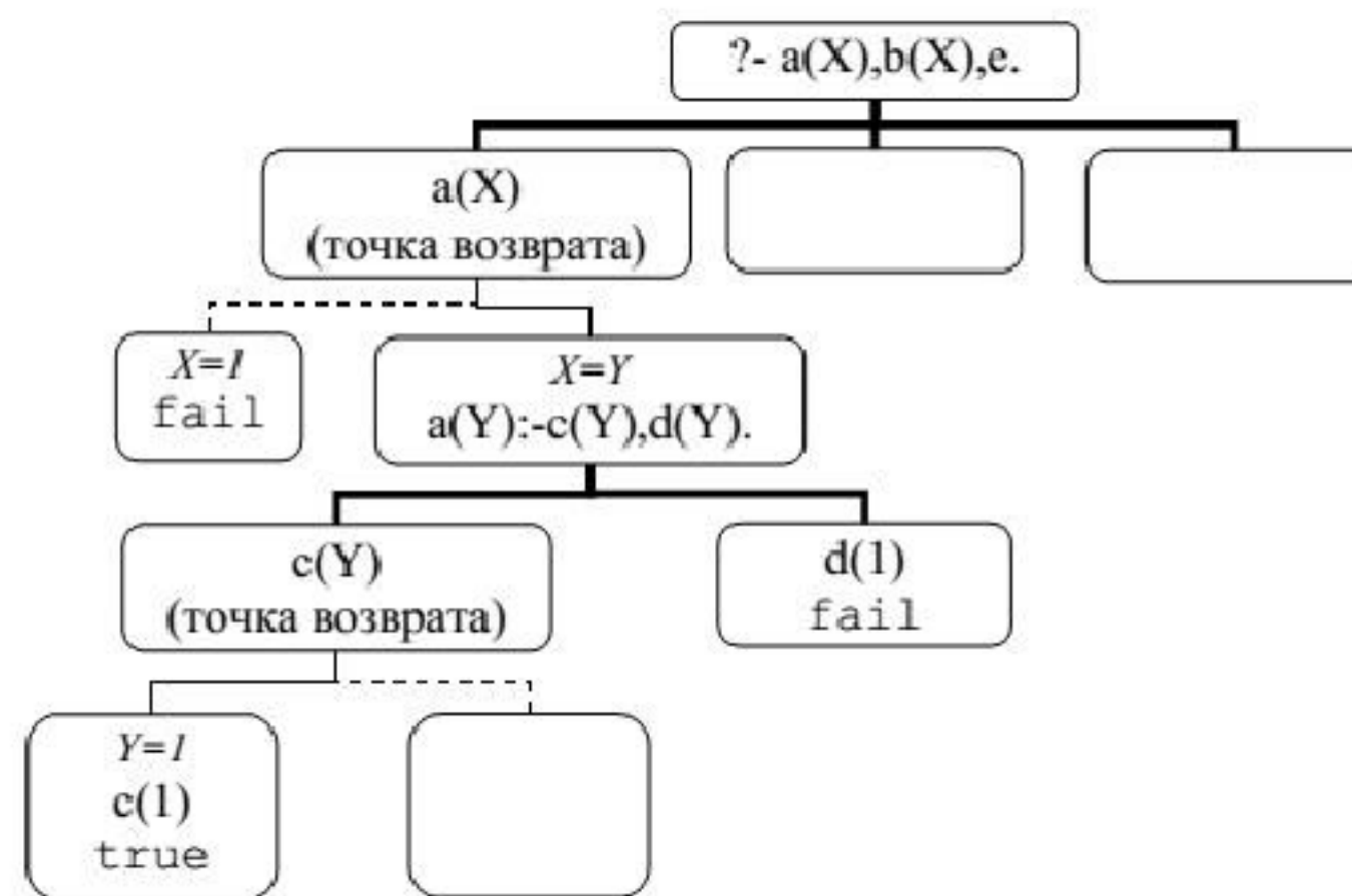
Рисунок 1.7 – Выполнение программы
