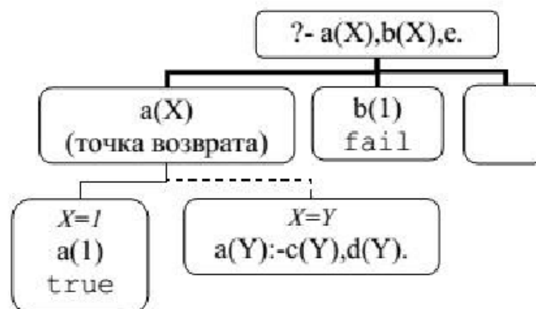
Рисунок 1.6 – Выполнение программы
