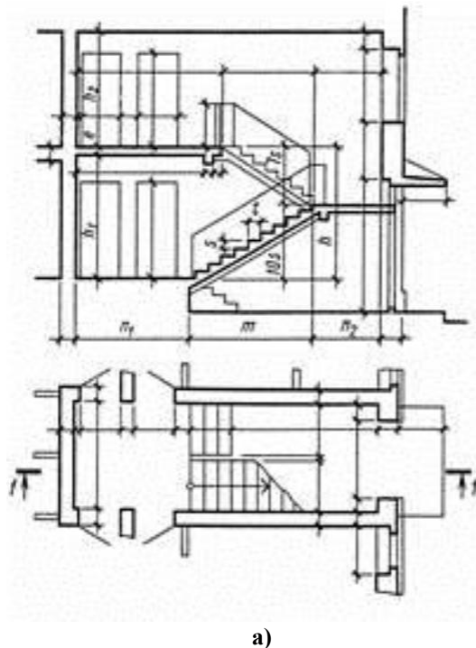
Рисунок 2 – Подготовки для обмеров а) лестничной клетки; б) плана здания.
