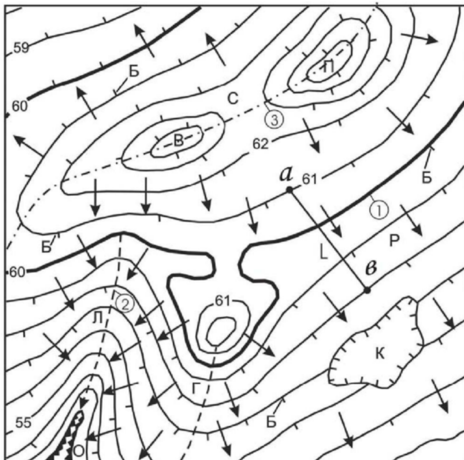
Рисунок 4 - Рельеф местности:
