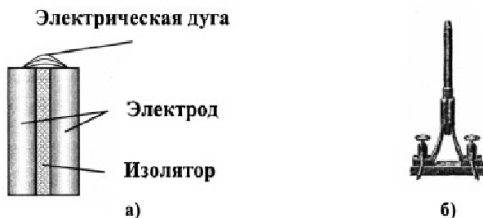
Рис. 4. Свеча Яблочкова
