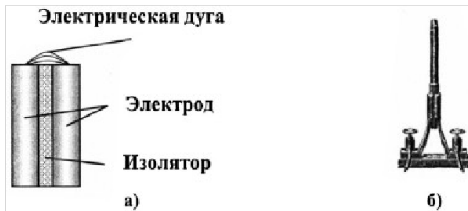
Рис. 4. Свеча Яблочкова
