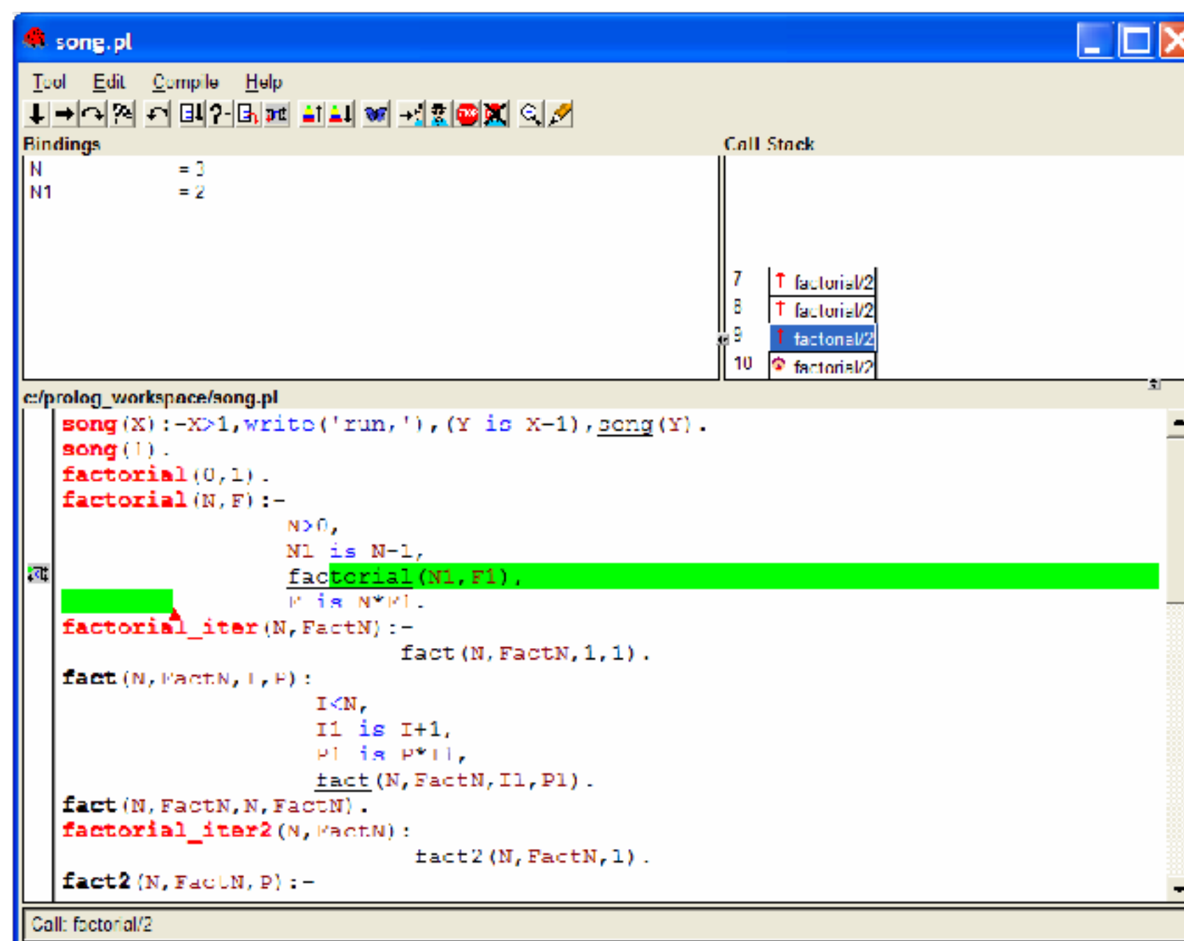
Рисунок 1.8 – Результат трассировки
