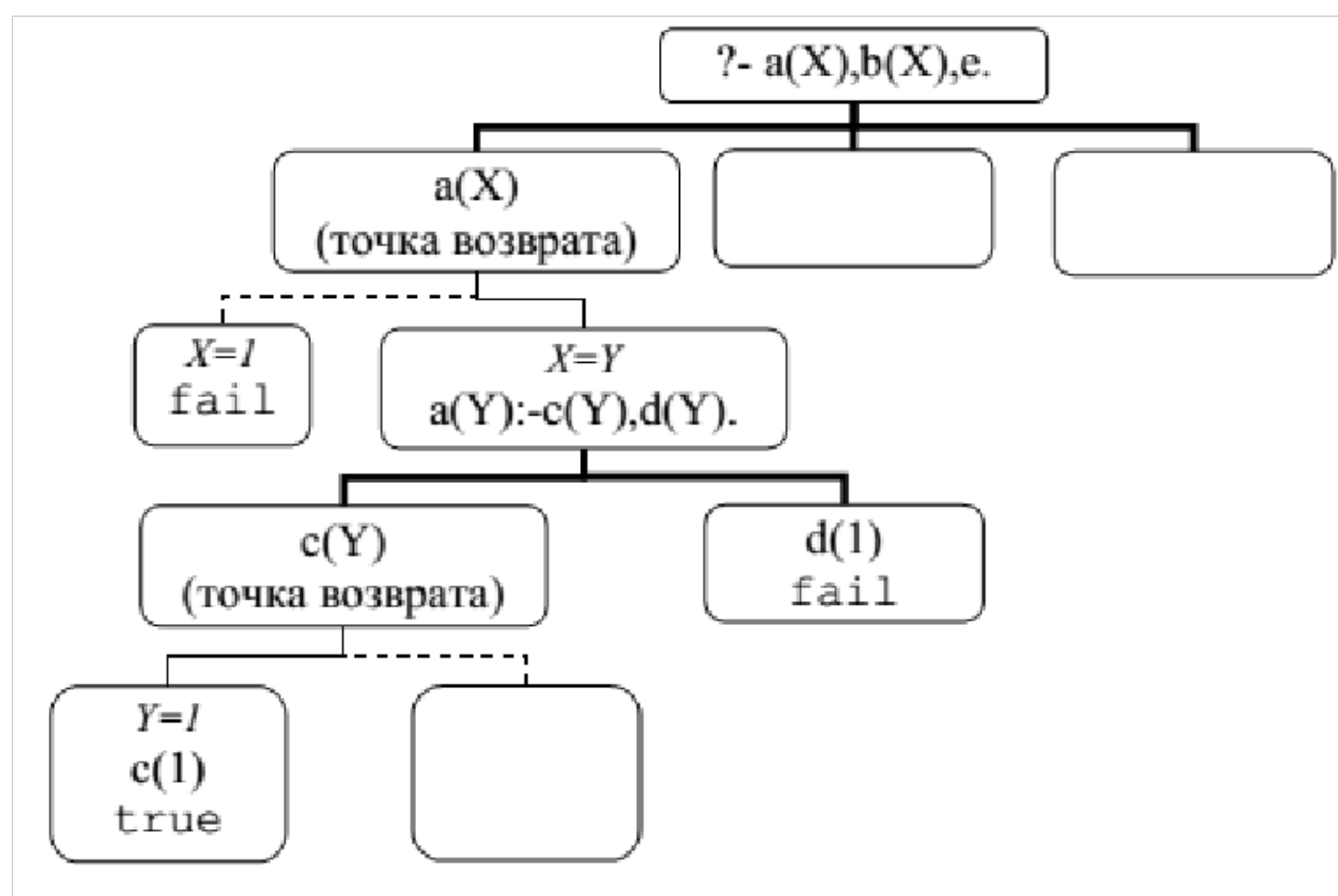
Рисунок 1.7 – Выполнение программы
