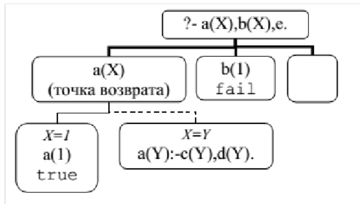
Рисунок 1.6 – Выполнение программы
