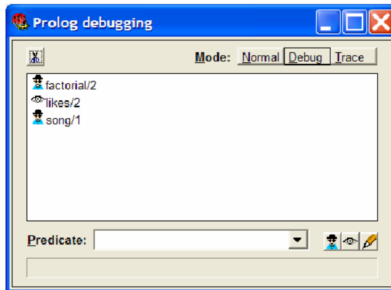
Рисунок 1.5 – Режим трассировки
