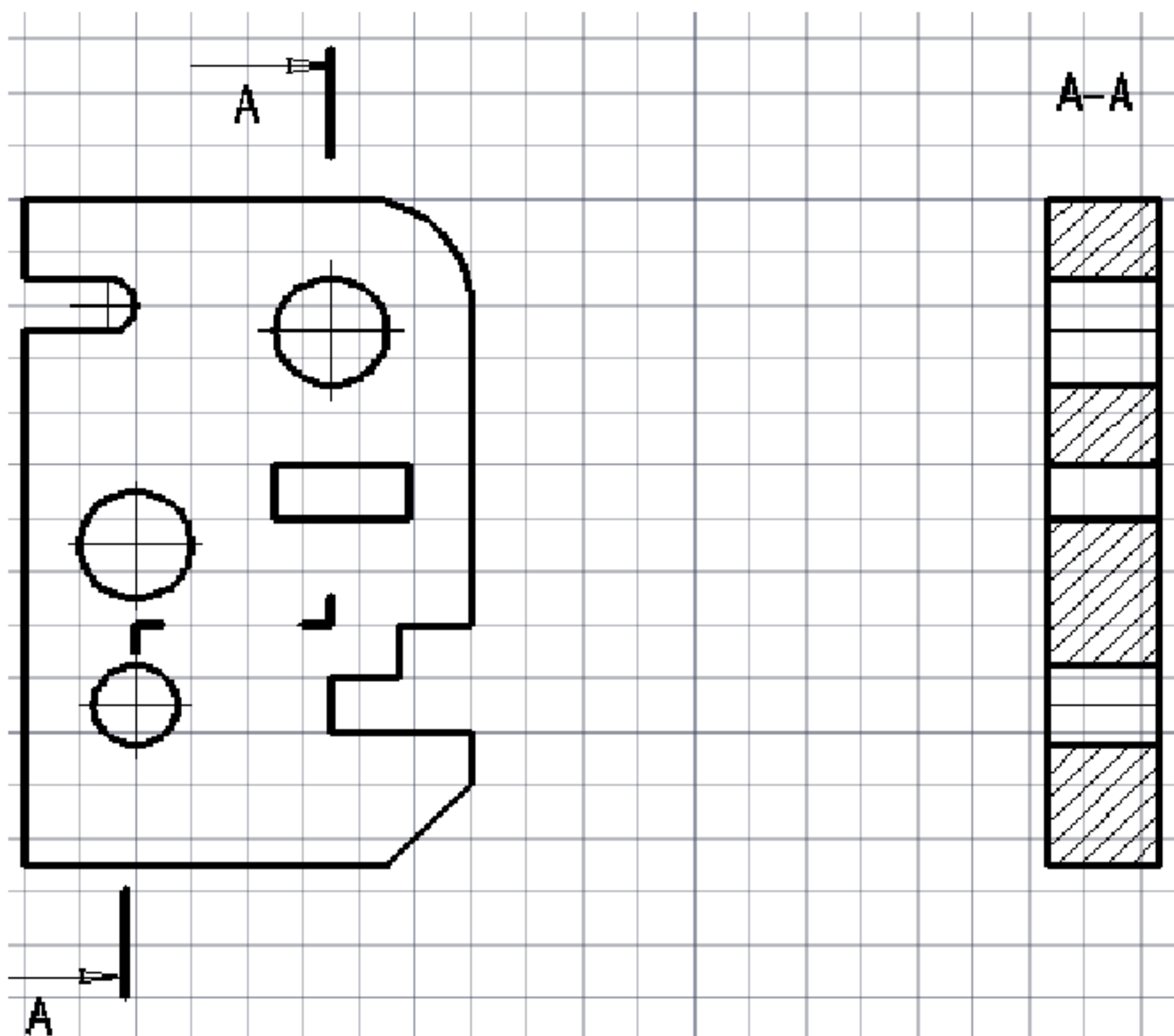
Рис. 2.12. Чертеж детали
