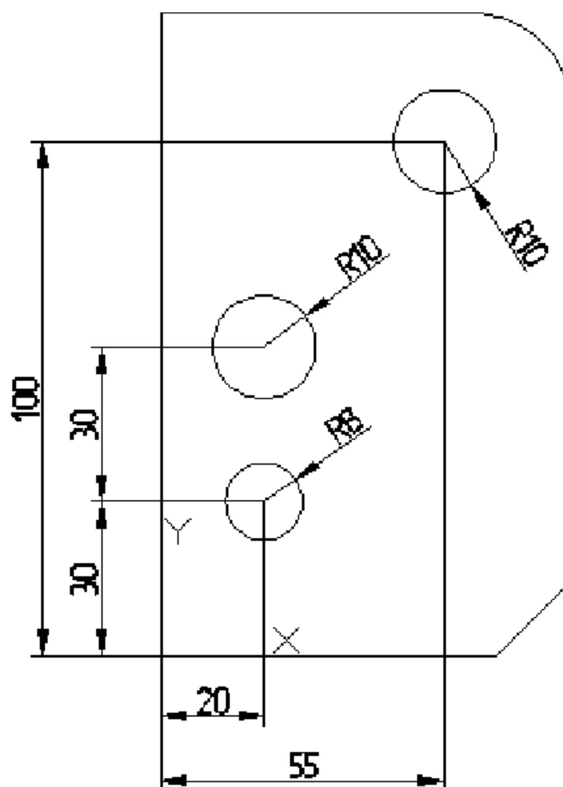
Рис. 2.3. Построение окружностей
