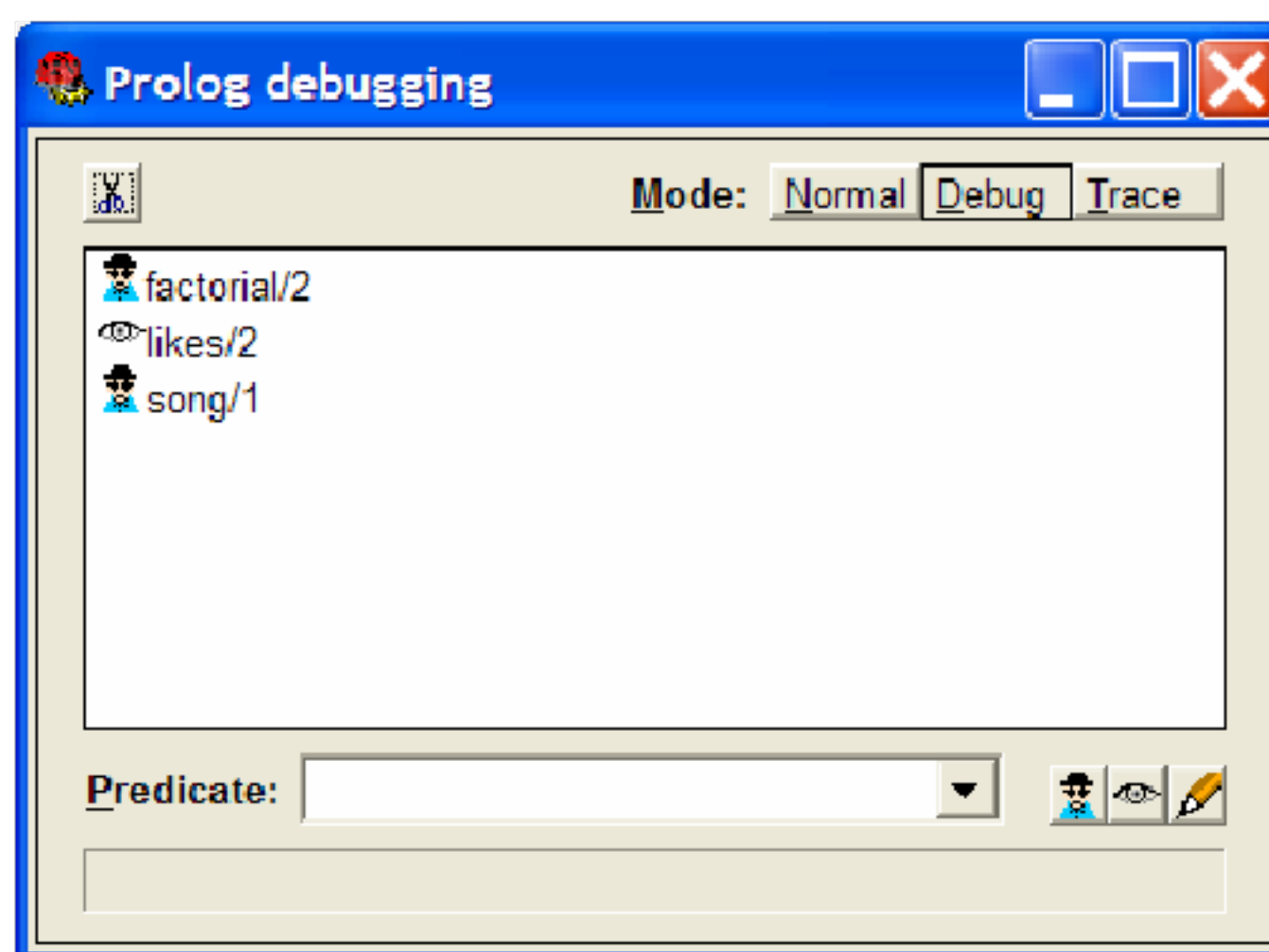
Рисунок 1.5 – Режим трассировки
