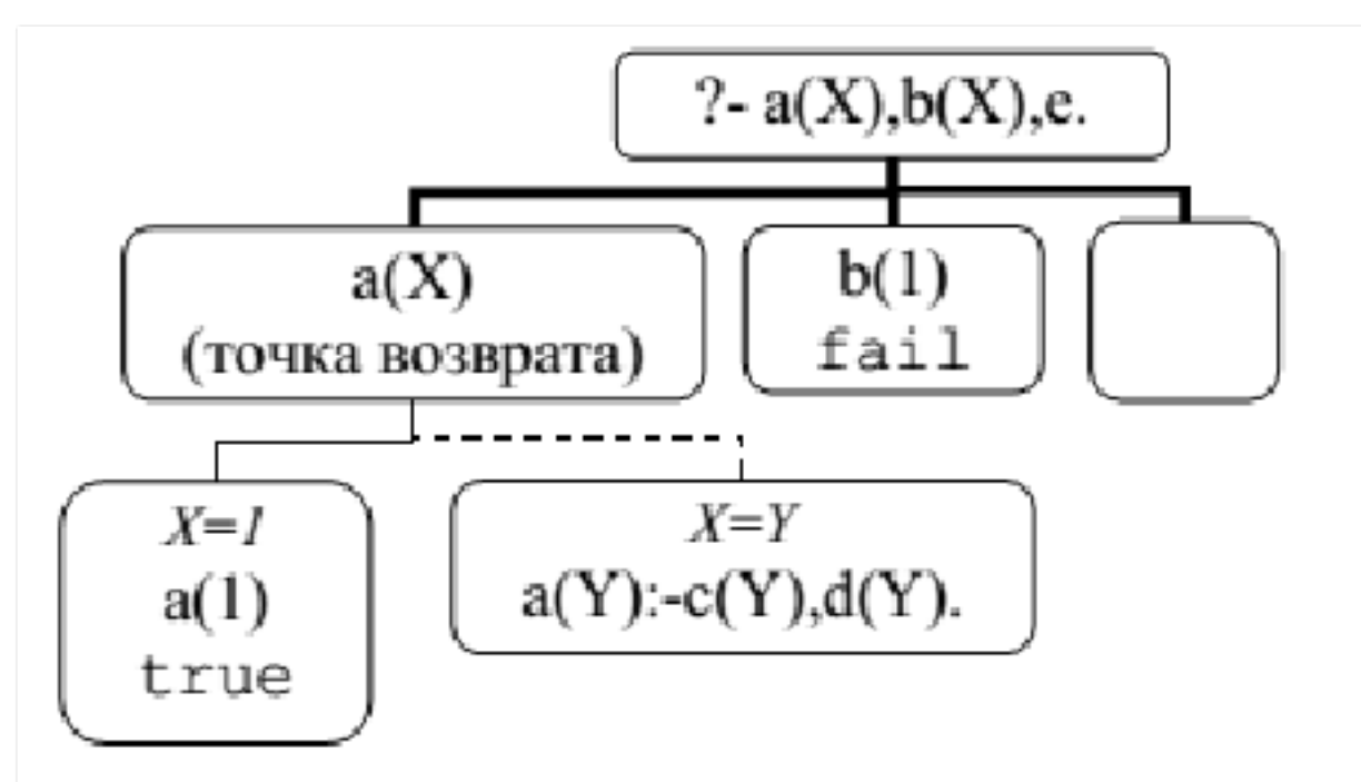
Рисунок 1.6 – Выполнение программы
