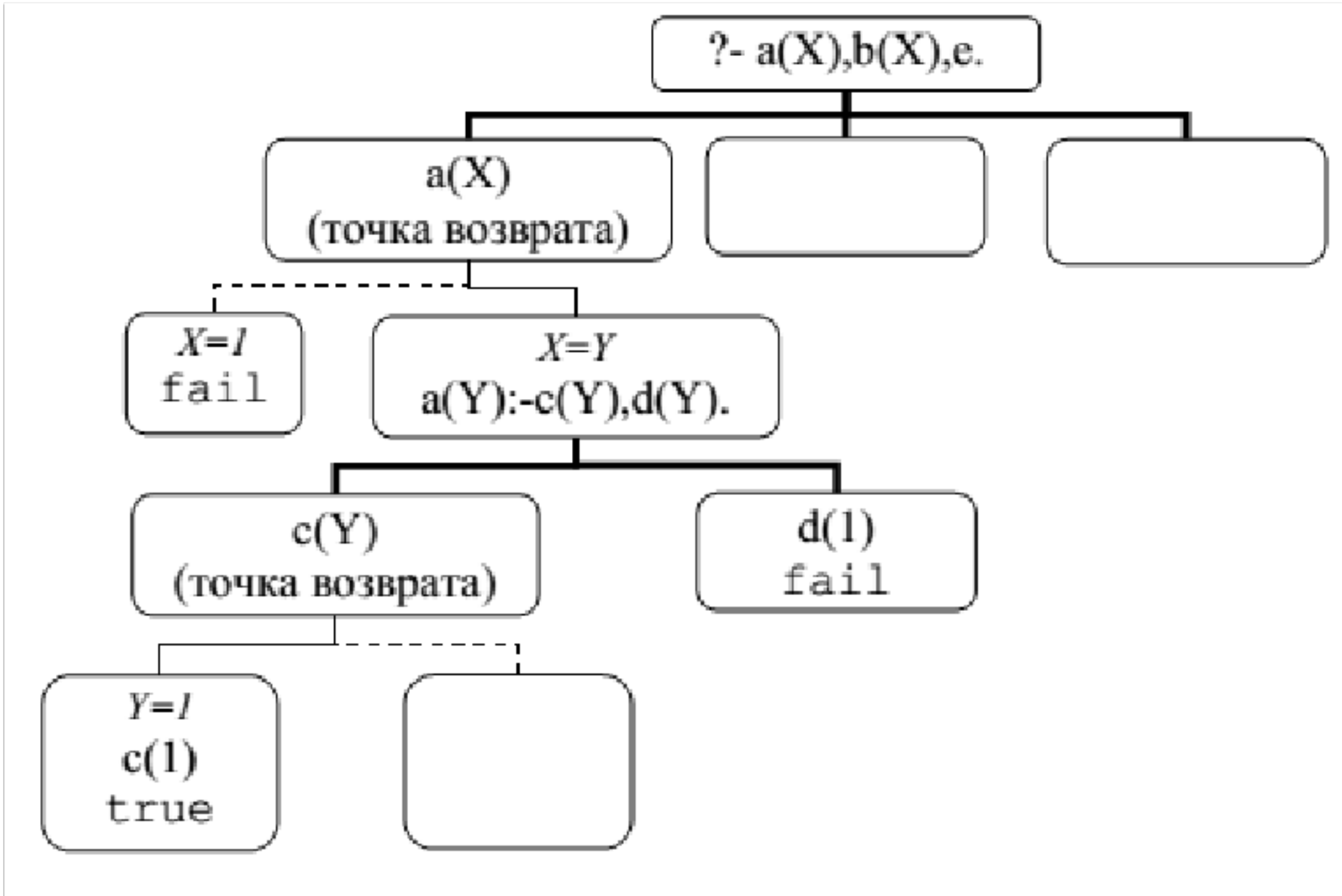
Рисунок 1.7 – Выполнение программы
