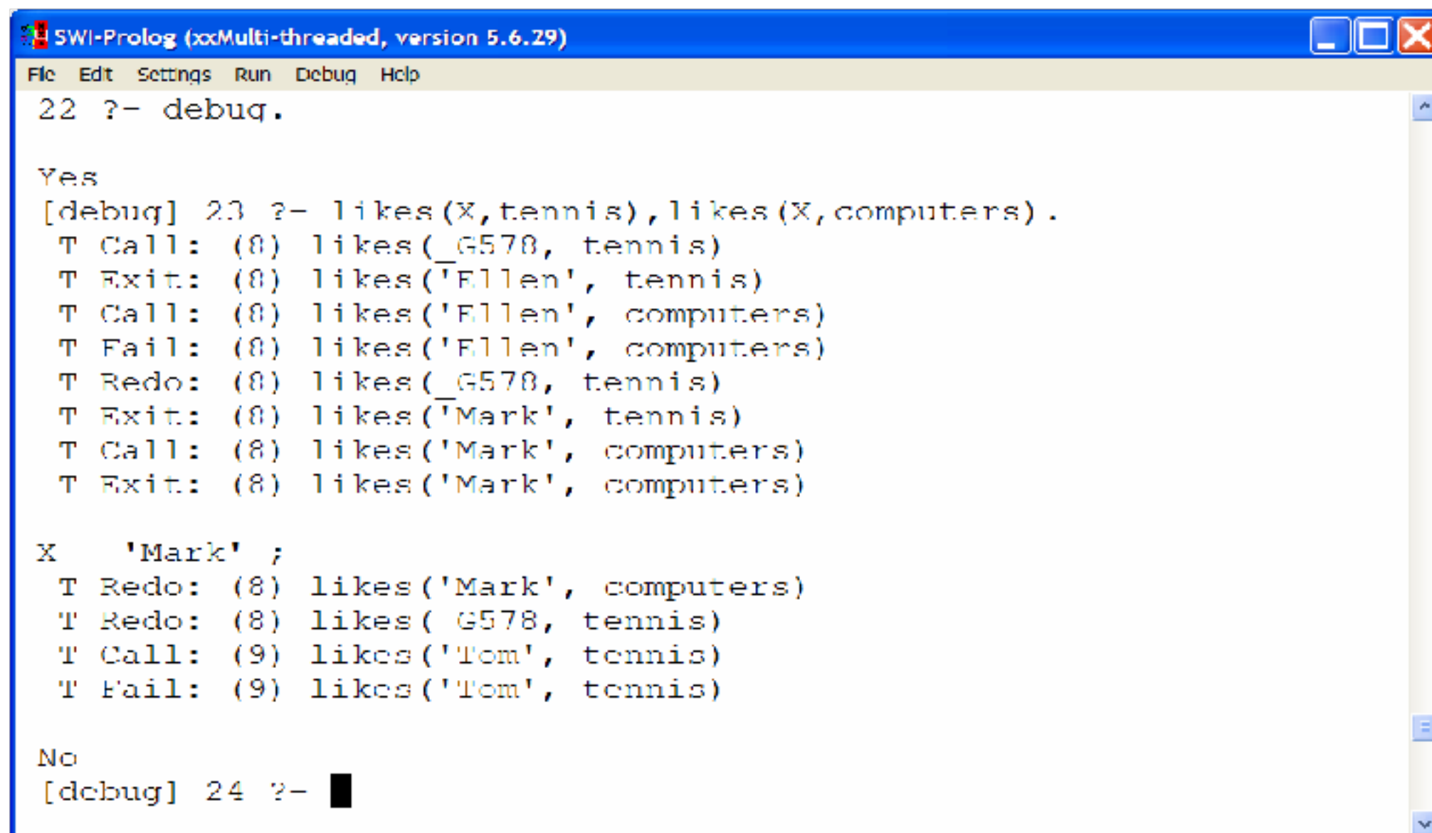
Рисунок 1.7 – Трассировка программы
