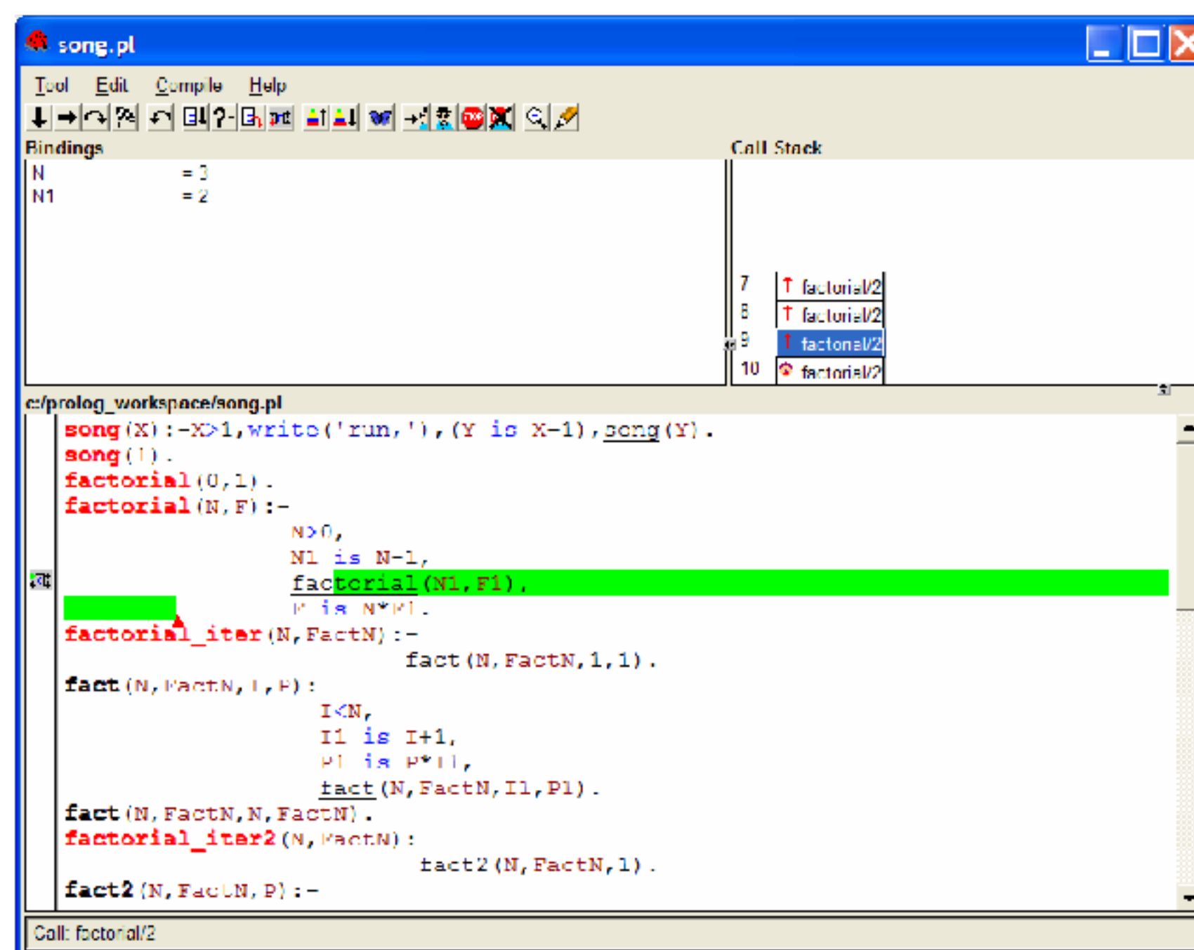
Рисунок 1.8 – Результат трассировки
