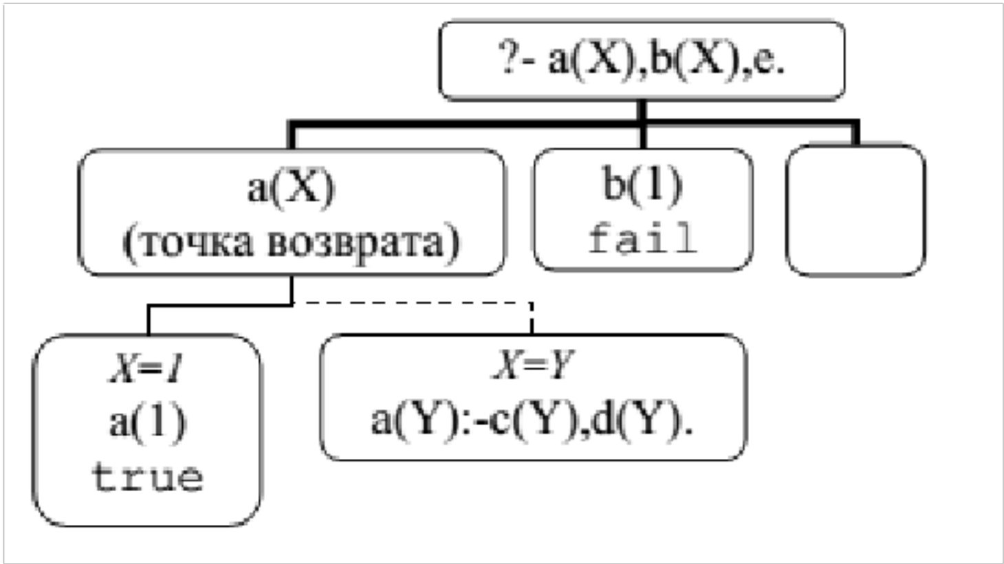
Рисунок 1.6 – Выполнение программы
