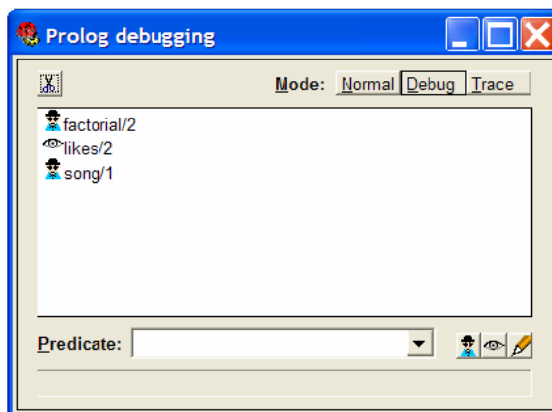
Рисунок 1.5 – Режим трассировки
