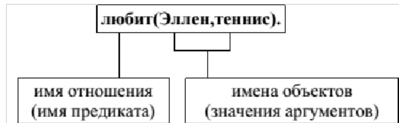
Рисунок 1.2 – Синтаксис Пролог
