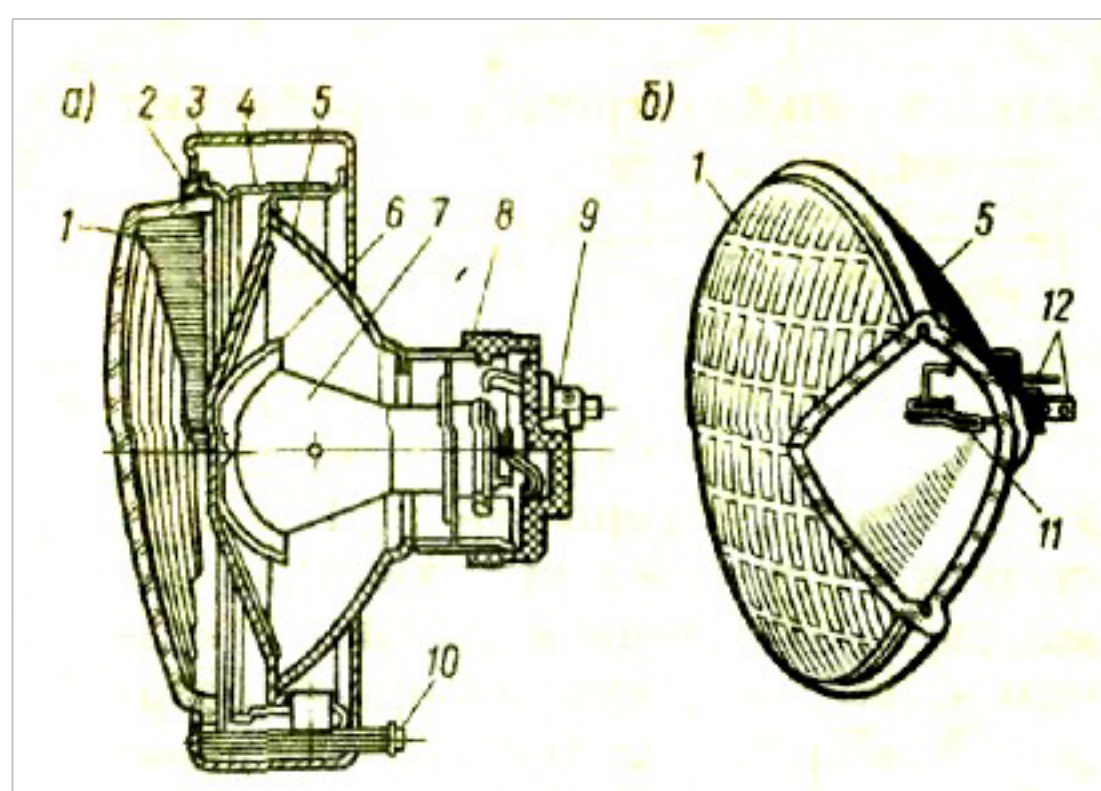
Рис. 4 - Специальные фары: а — противотуманная фара, б - лампа-фара; 1 — рассеиватель, 2—резиновая прокладка; 3 — ободок. 4 — установочное кольцо, 5— рефлекс, 6 — экран с держателем; 7 — лампа, 8 — патрон. 9 — вывод пружинящего контакта; 10 — винт для регулировки фары. 11 — вольфрамовые спирали. 12— выводы спиралей
