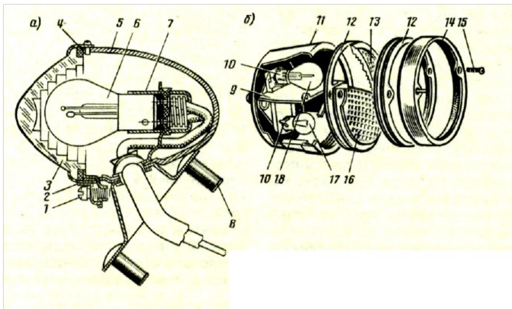
Рис. 5 - Подфарник и задний фонарь
