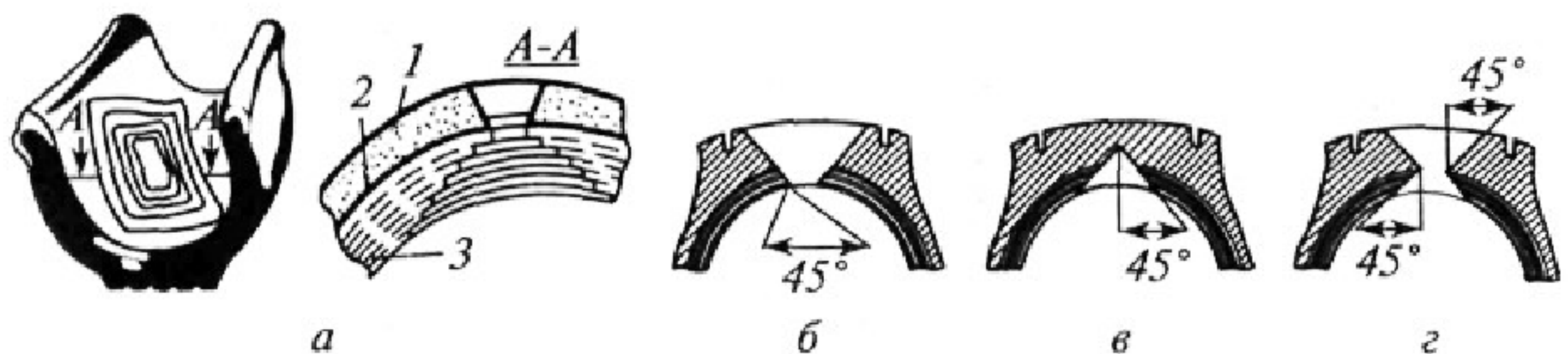
Рис. 5.1. Способы вырезки поврежденных участков покрышки:
