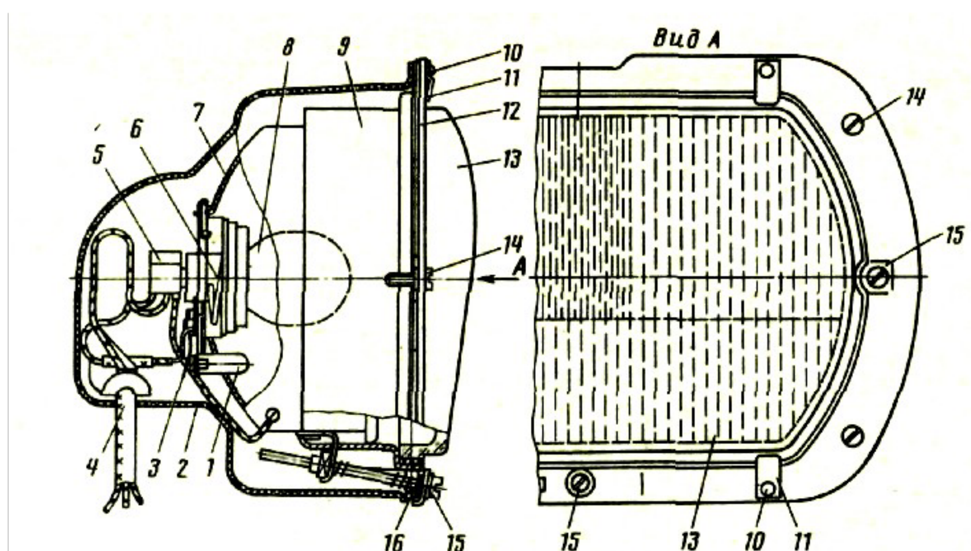
Рис. 8.3 Прямоугольная фара
