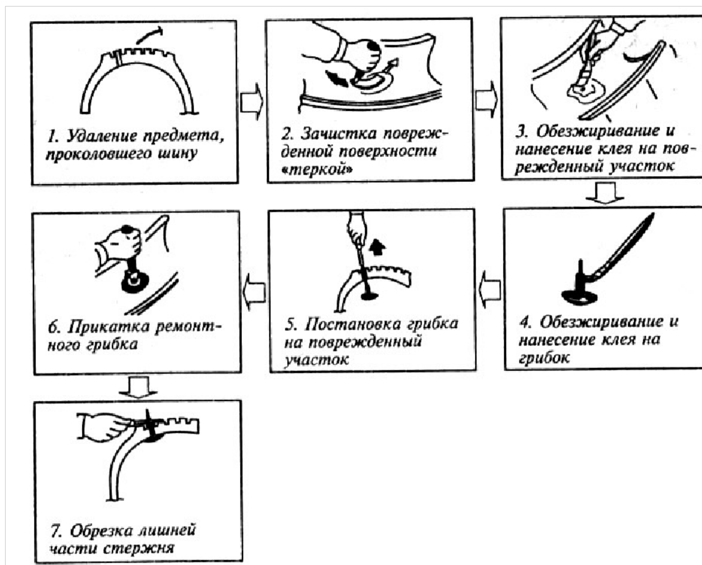
Рис. 5.5. Технология ремонта бескамерной шины с использованием автоаптечки
