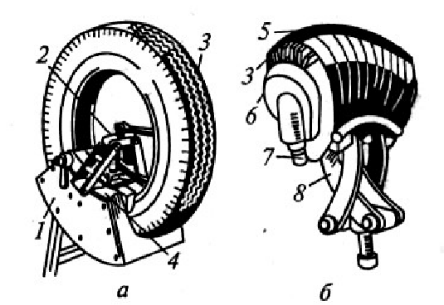
Рис. 5.6. Аппараты для вулканизации покрышек:
