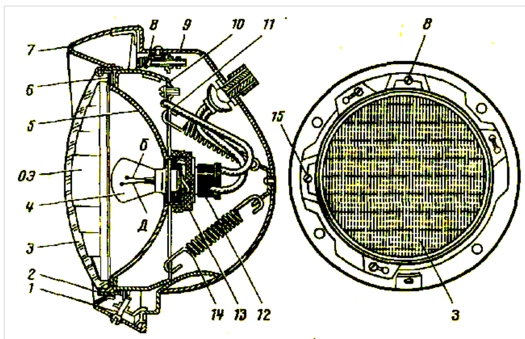
Рис. 2 - Круглая фара
