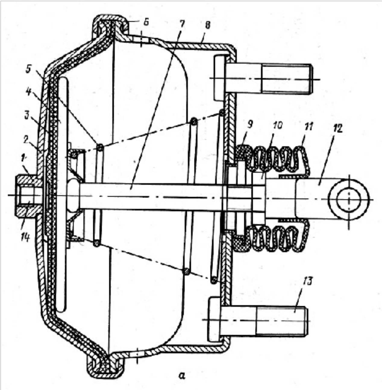
Рис. 5 - Тормозные камеры пневматической системы тормозов автомобиля: а
