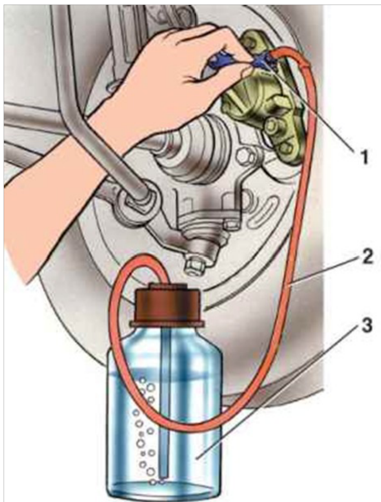
Рисунок 1. Прокачка рабочего тормозного цилиндра: 1 – рабочий тормозной цилиндр; 2 – гибкая прозрачная трубка; 3 – ёмкость с тормозной жидкостью.
