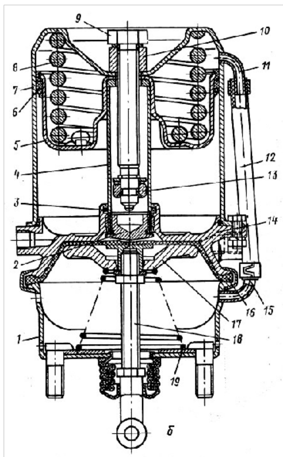
Рис. 5, б - Тормозная камера задней тележки:
