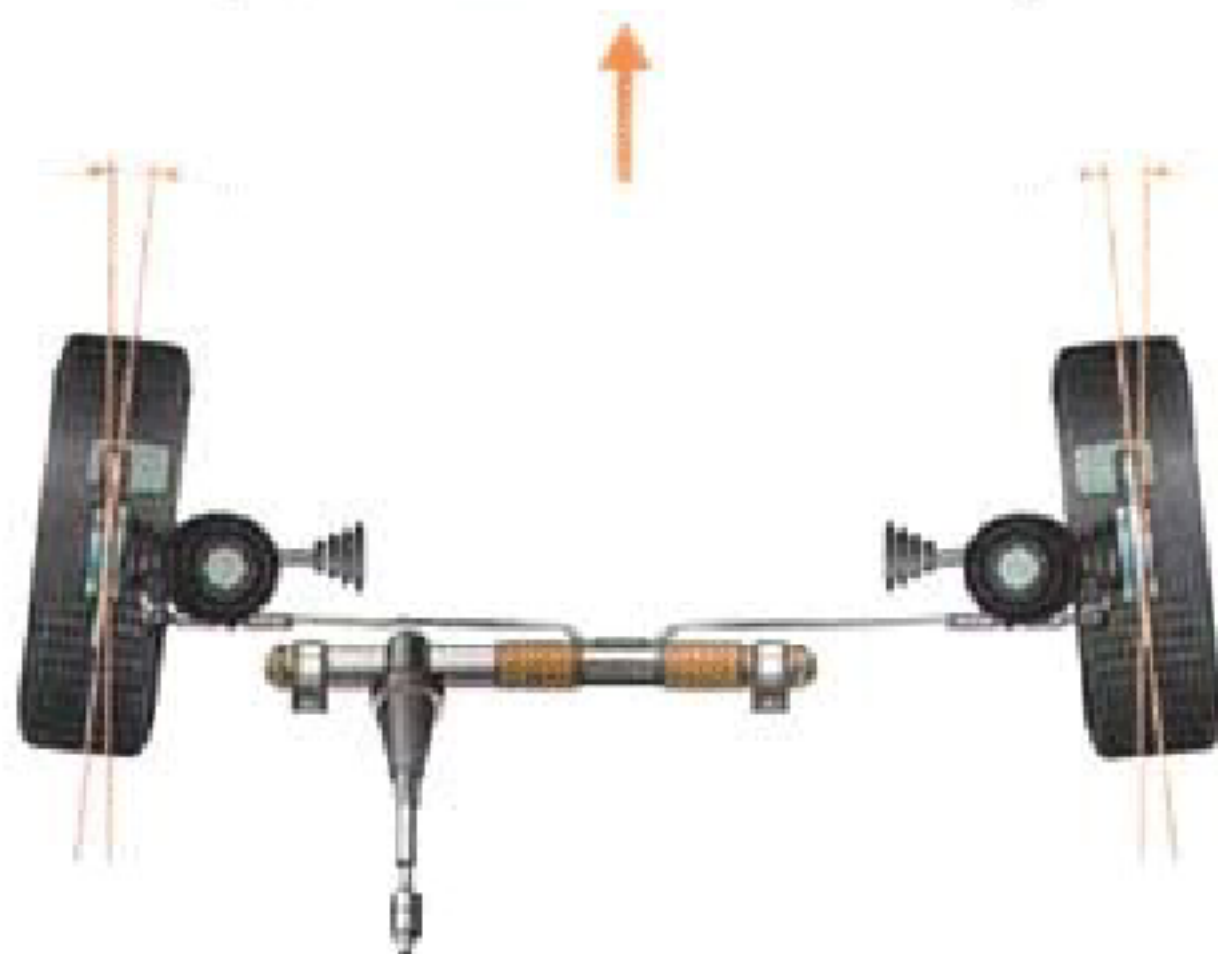
Рис. 3. Схождение колес.
