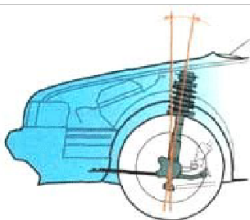
Рис. 1. Угол продольного наклона оси поворота колеса.
