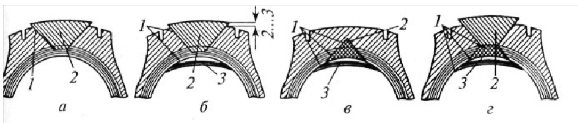
Рис. 5.3. Заделка повреждений при вырезке участка способами: а и б — наружным конусом; в — внутренним конусом; г — встречным конусом; 1 — прослоечная резина; 2 — протекторная резина; 3 — пластырь
