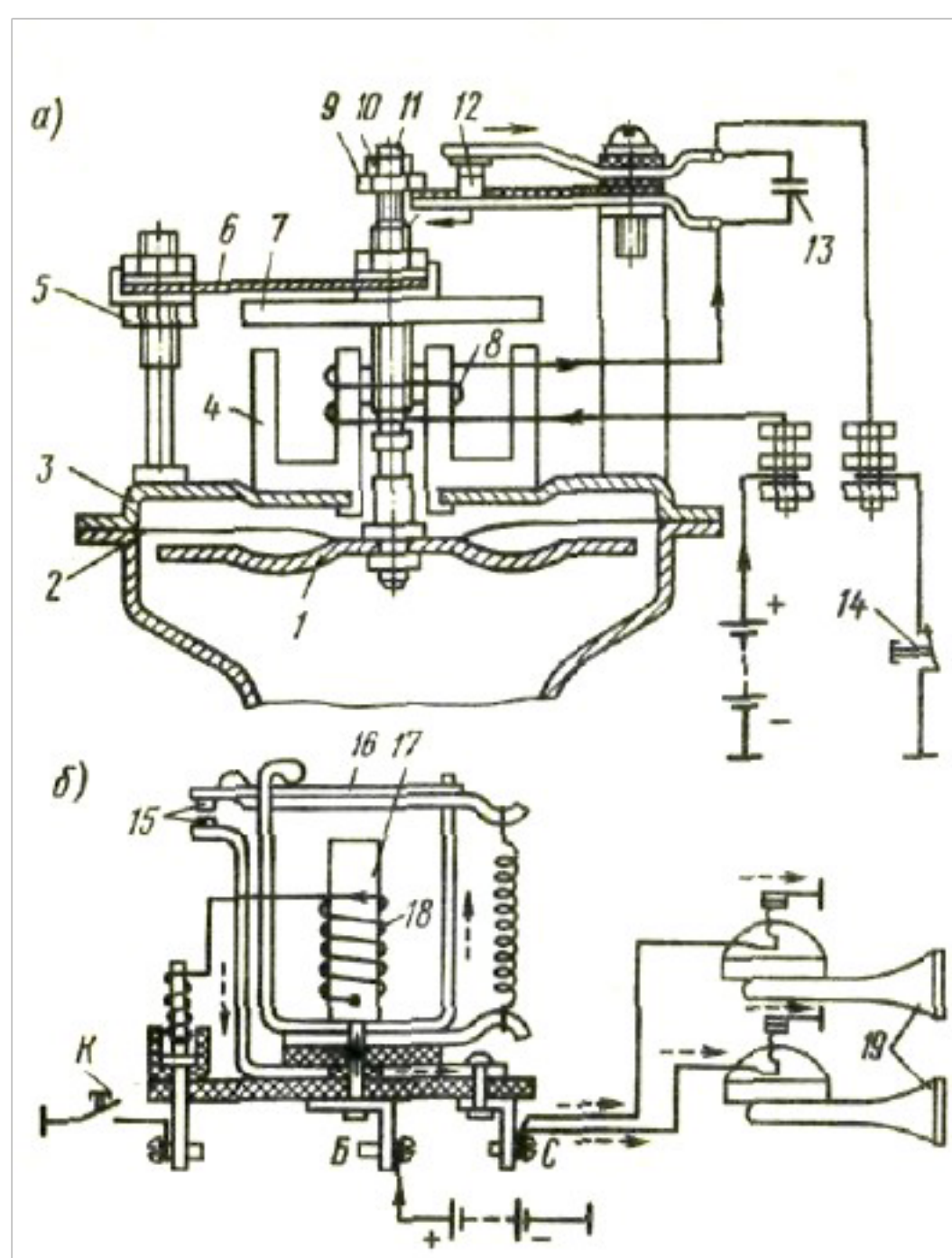
Рис. 7 - Звуковой сигнал: а — схема звукового сигнала, б — схема реле сигналов
