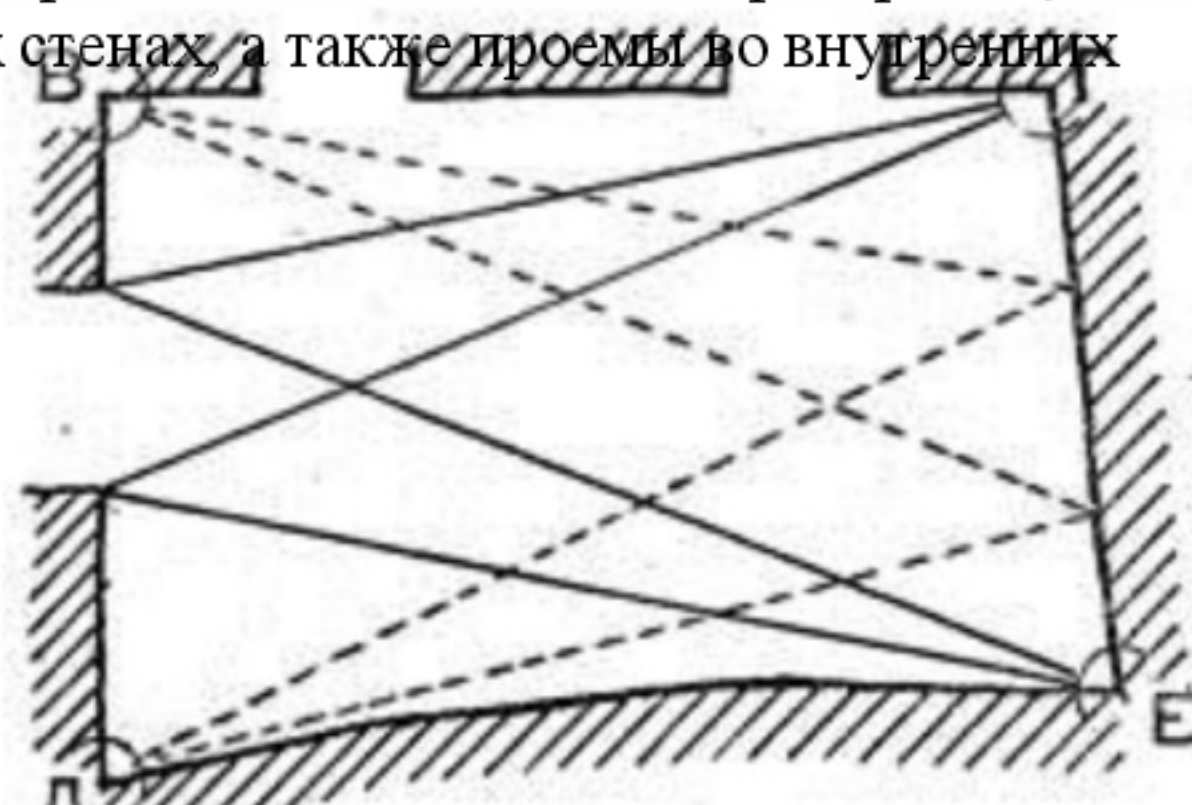
Рисунок 4а триангуляционная система обмеров
