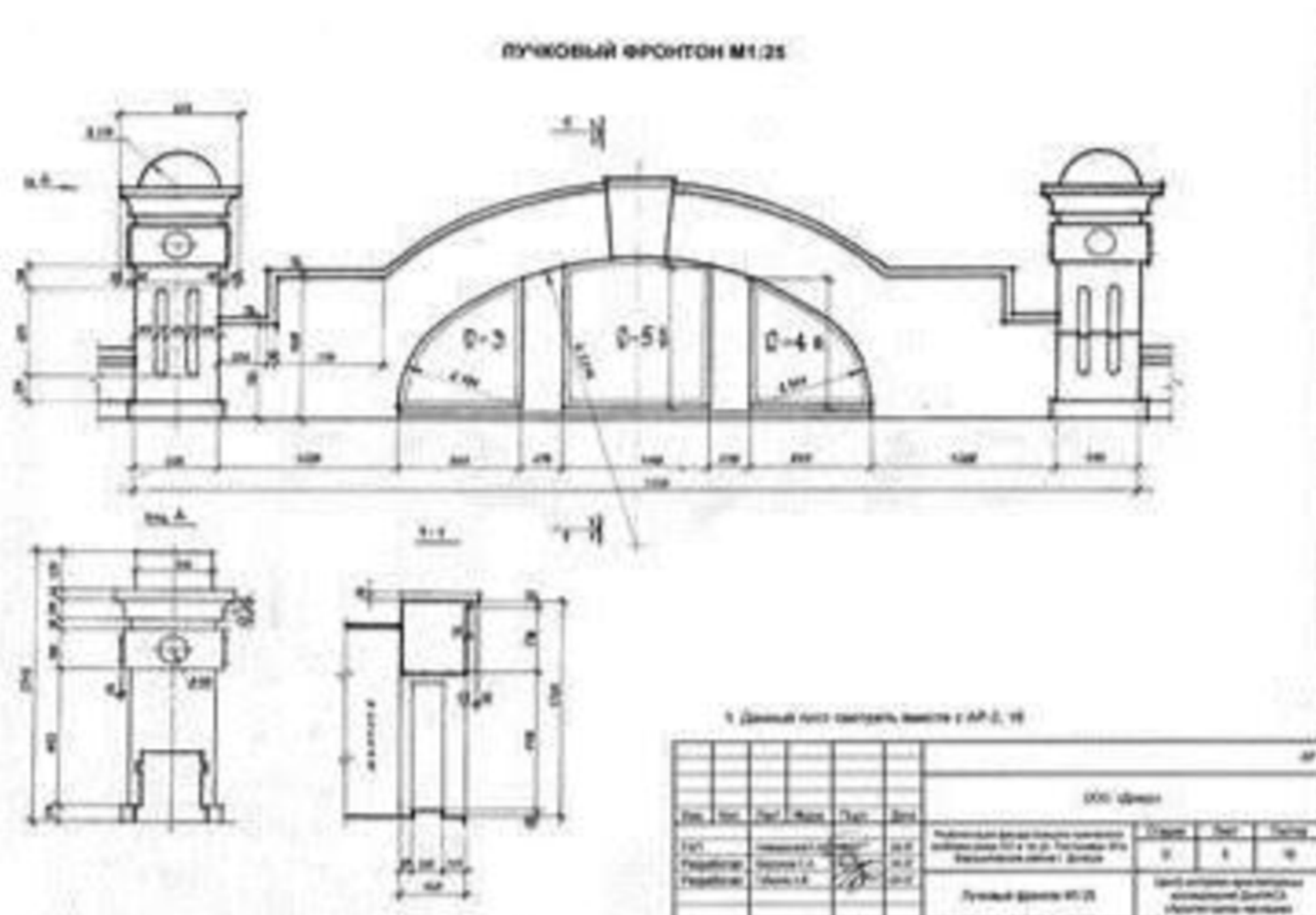
Рисунок 5 – Обмеры деталей: подробный обмер лучкового фронтона
