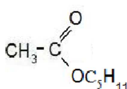
изоамилацетат
