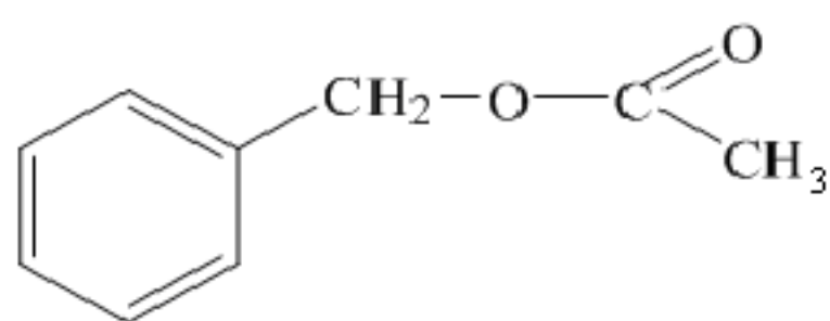
бензилацетат
