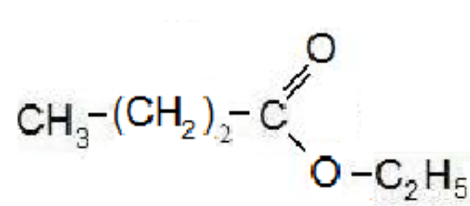
этилбутират
