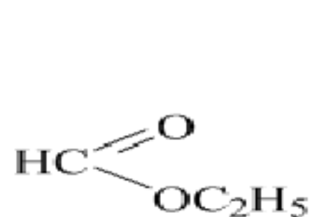
этилформиат
