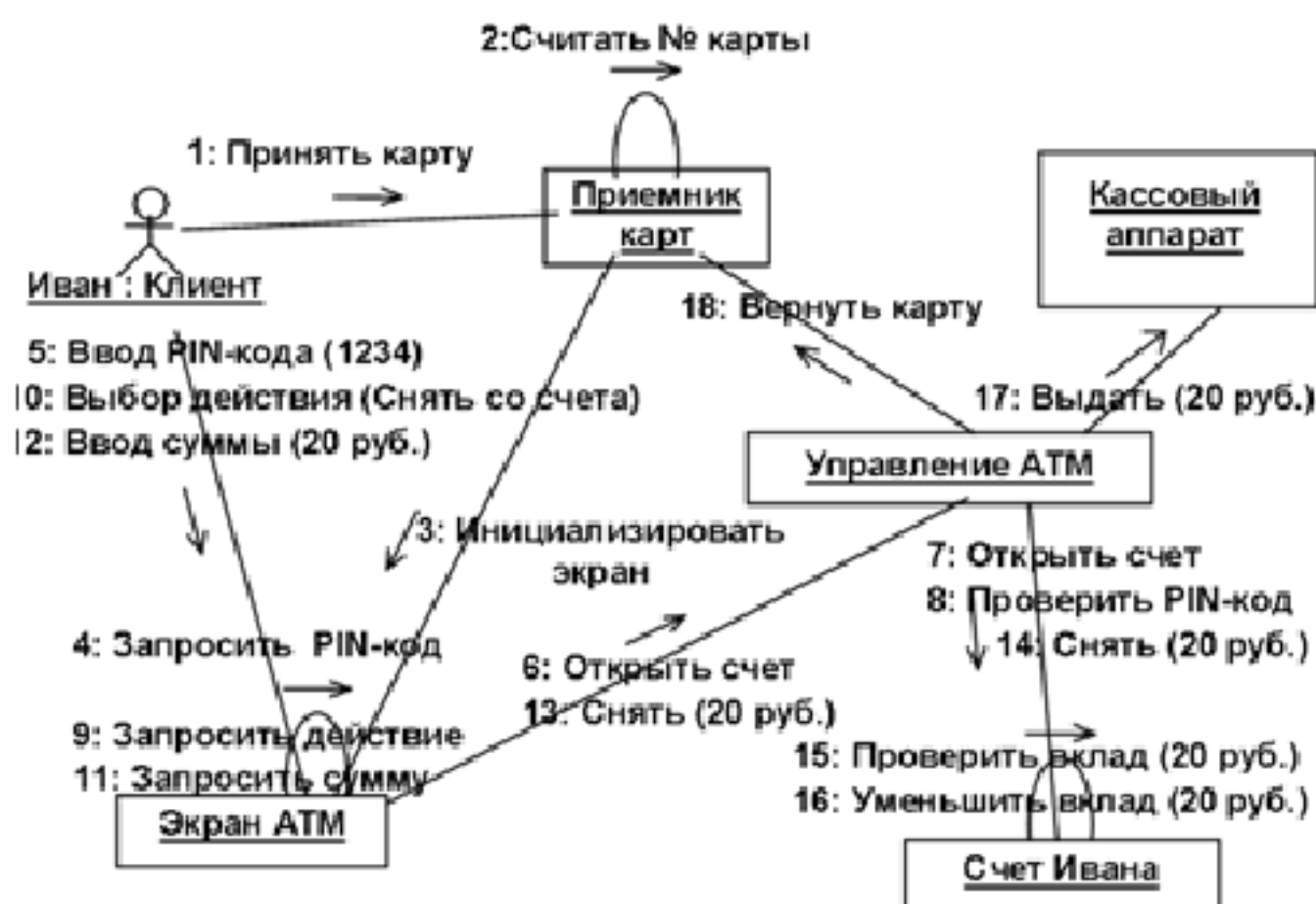
Рисунок 3.8 - Пример диаграммы кооперации
