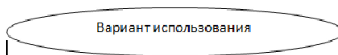
Рисунок 3.2 - Вариант использования
