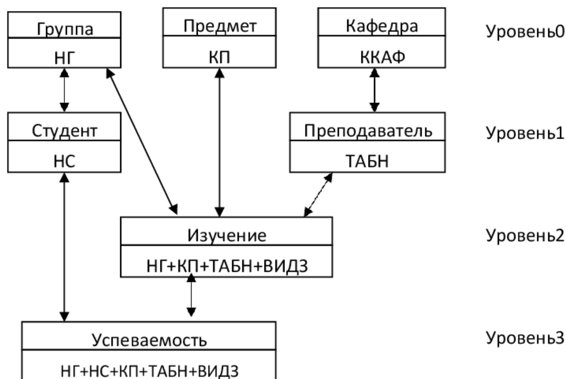
Рисунок 7.6 Информационно-логическая модель предметной области "Учебный процесс"
