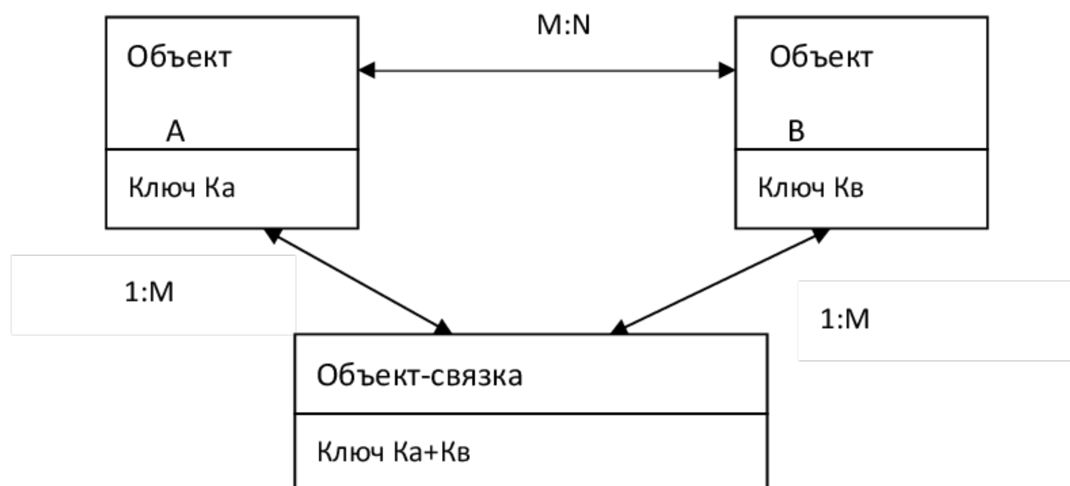
Рисунок 7.5 - Преобразование связи типа M:N через объект-связку.
