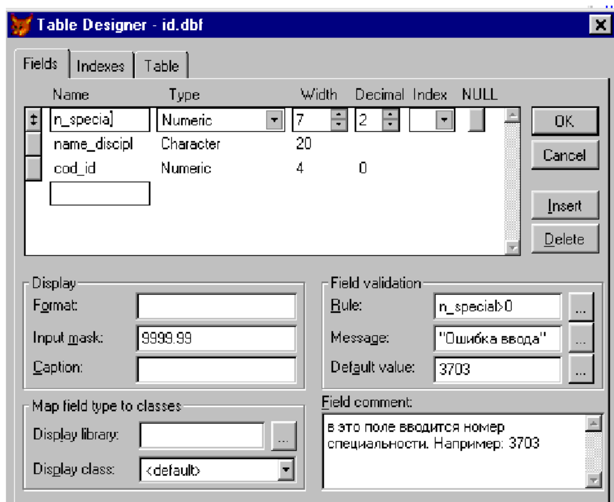
Рисунок 3 - Вкладка Fields Конструктора таблиц с дополнительными областями.
