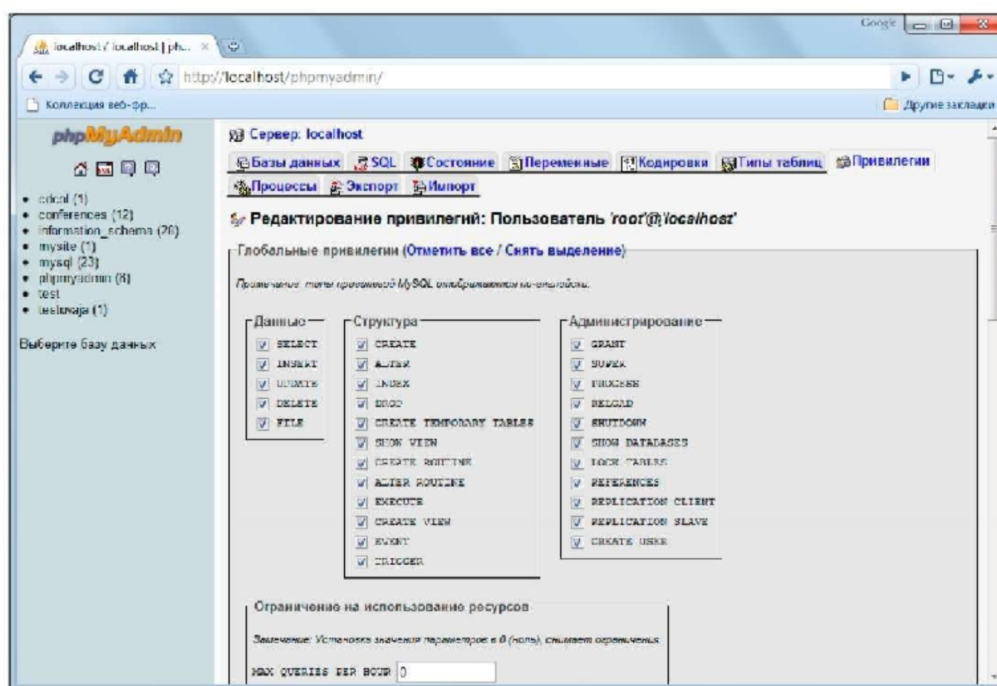
Рисунок 4. Интерфейс страницы для редактирования данных учетной записи
