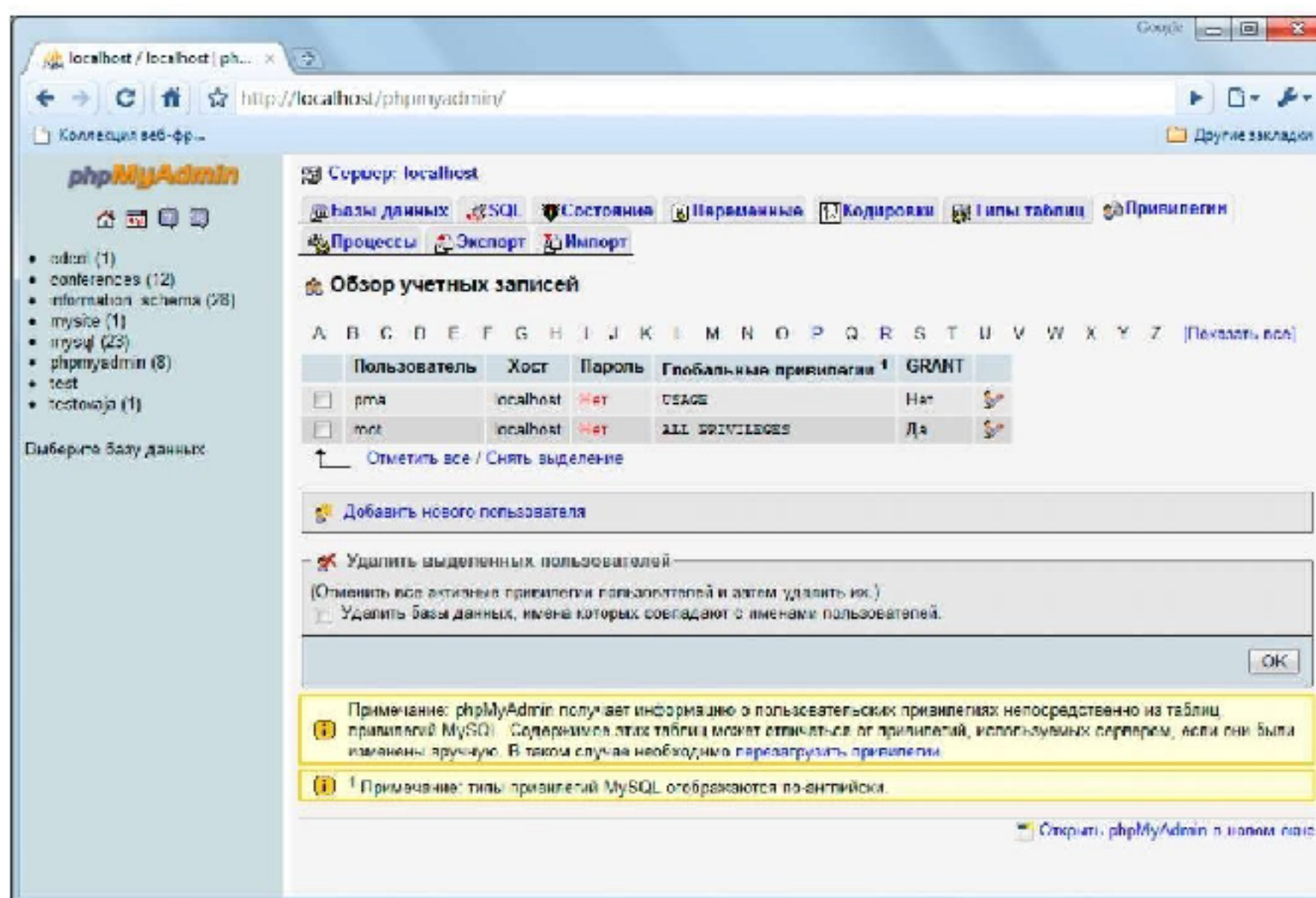
Рисунок 2. Интерфейс вкладки «Привилегии» системы phpmyadmin
