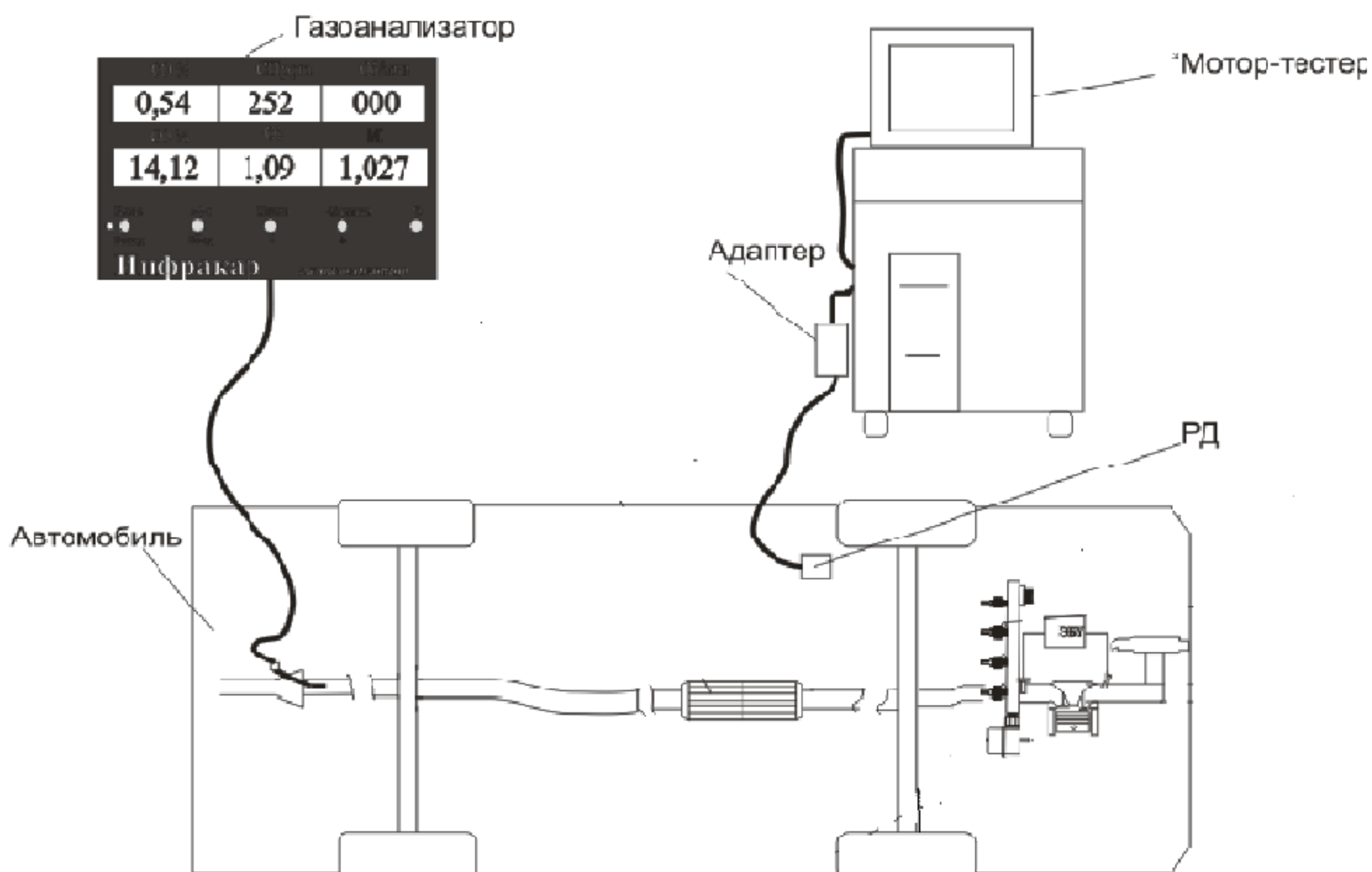
Рис. 12. Экспериментальная установка.
