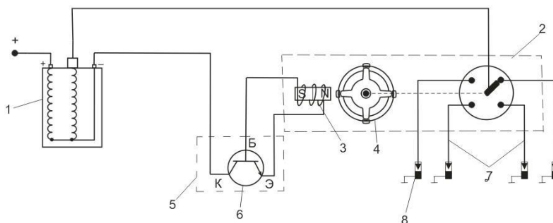
Рис. 13. Принципиальная электрическая схема транзисторной системы зажигания с индукционным датчиком: 1-катушка зажигания; 2-распределитель; 3-индукционный датчик; 4-зубчатый ротор; 5-коммутатор; 6-транзистор; 7-высоковольтные провода; 8-свечи зажигания
