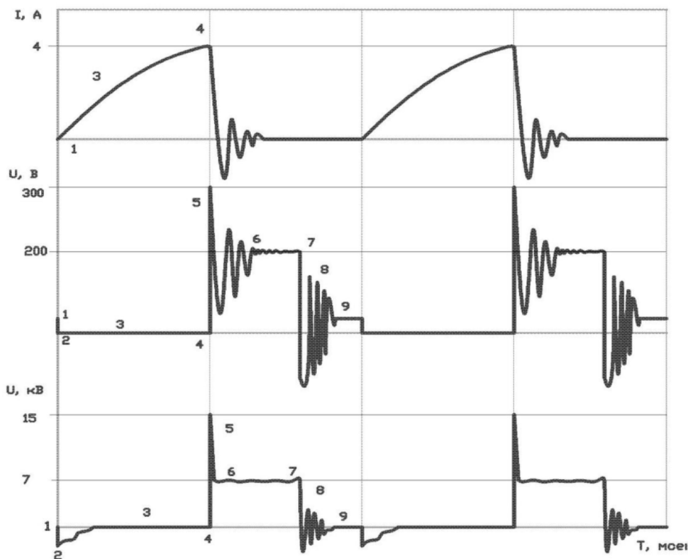
Рис. 4. Осциллограммы первичной и вторичной обмоток катушки зажигания
