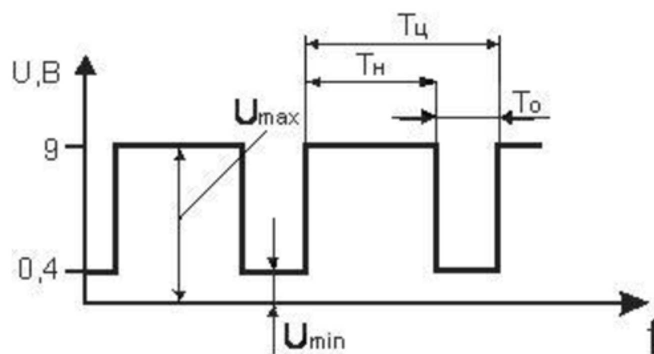
Рис. 2. Осциллограмма импульсного сигнала: U_{max} , U_{min} – максимальное и минимальное значение напряжения; T_H – время действия сигнала (поддержания U_{max} ); T_0 – время поддержания U_{min} ; T_C – время цикла
