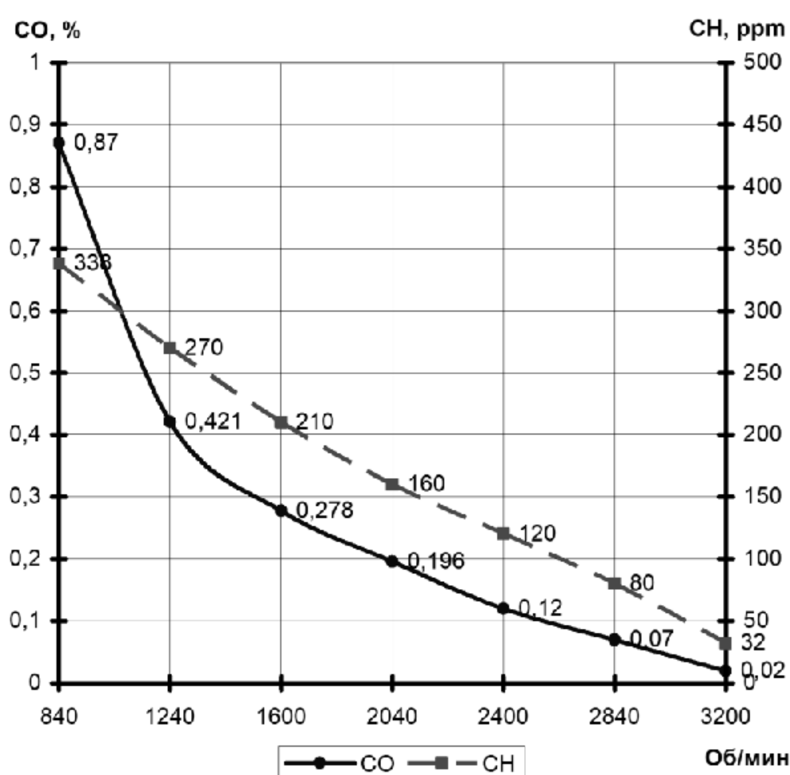
Рис. 15 Зависимость содержания \text{CO} и \text{CH} от частоты вращения коленчатого двигателя.
