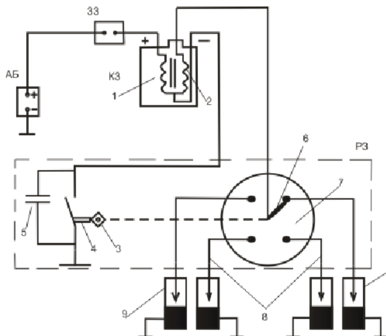
Рис. 5. Электрическая схема контактной системы зажигания.
