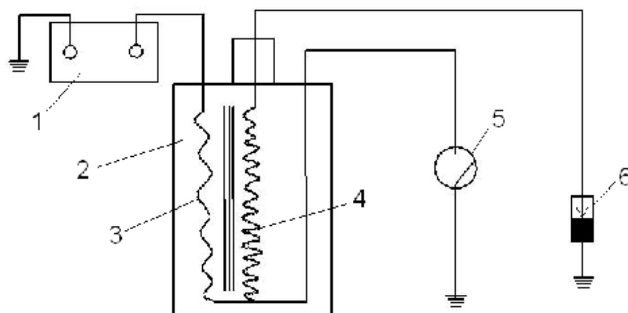
Рис. 3 Система зажигания: 1-аккумулятор; 2-катушка зажигания; 3-первичная обмотка катушки зажигания; 4-вторичная обмотка катушки зажигания; 5-лампочка; 6-датчик Холла.
