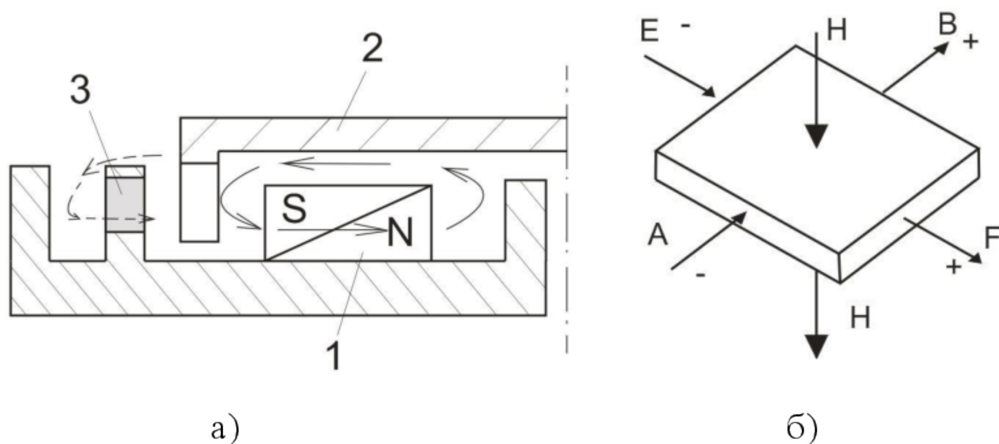
Рис. 7. Схема датчика импульсов напряжений (датчик Холла)
