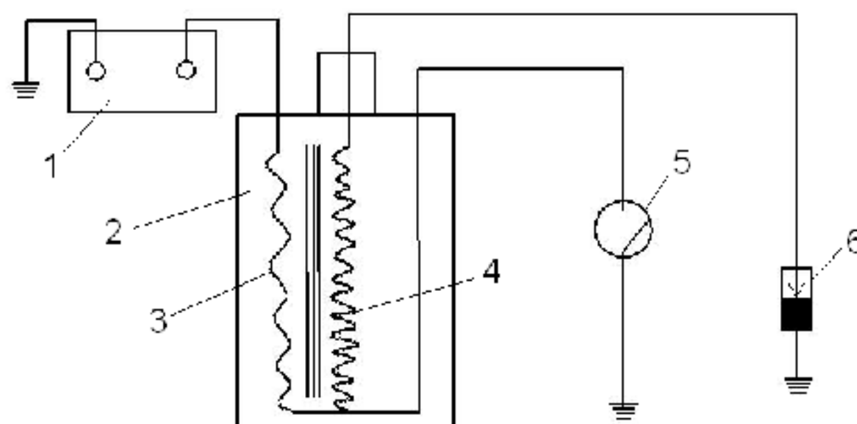
Рис. 3 Система зажигания: 1-аккумулятор; 2-катушка зажигания; 3-первичная обмотка катушки зажигания; 4-вторичная обмотка катушки зажигания; 5-лампа; 6-датчик Холла.
