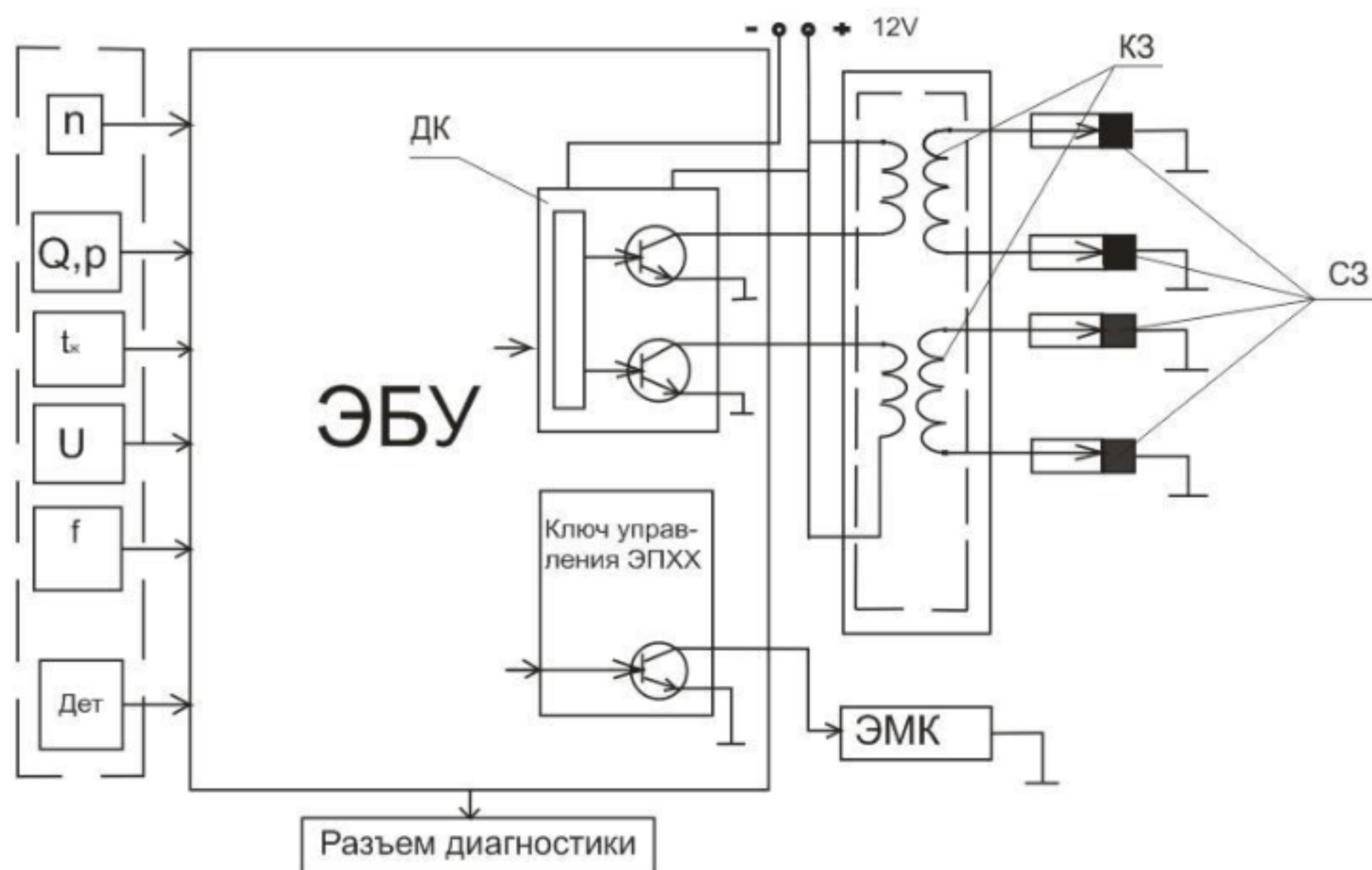
Рис. 14 Блок-схема микропроцессорной системы зажигания: n – датчик частоты вращения коленчатого вала; Q, P – датчик нагрузки на охлаждающей жидкости; U – сигнал датчика детонации; f – конечный датчик
