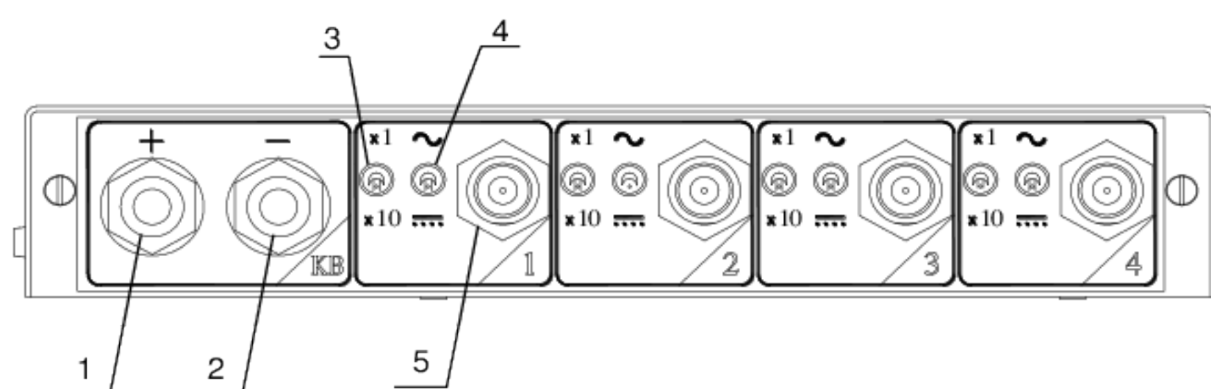
Рис. 21. Модуль обработки сигналов: 1,2- разъемы для подключения датчиков высокого напряжения положительной и отрицательной полярности; 3-индикатор питания; 4-переключатель диапазона измеряемого напряжения; 4-тумблер
