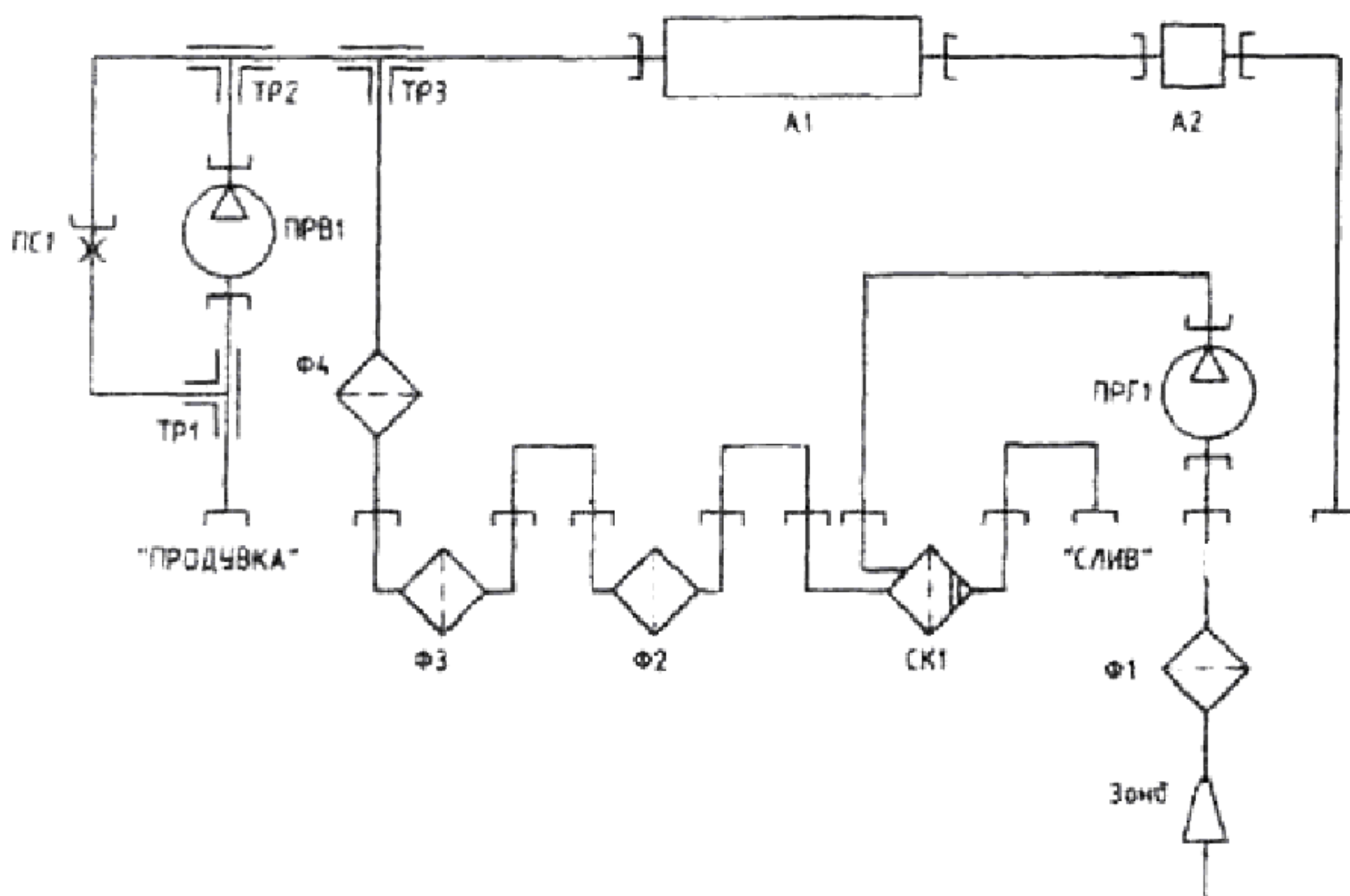
Рис. 1. Схема пневматическая: Φ1 – бензиновый фильтр, ПРГ1 - насос выхлопных газов, СК1- каплеотбойник, Φ2, Φ3, Φ4 – фильтры тонкой очистки, А1 – кювета, А2 – датчик кислорода: ПРВ1 – насос продувки воздухом, РС1 – пневмосопротивление, ТР1, ТР2, ТР3 – тройники.
