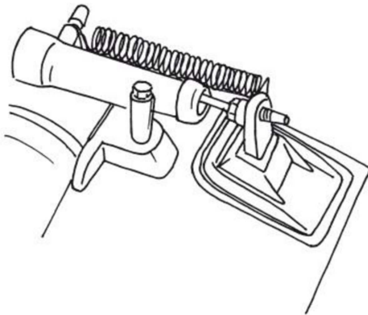
Рисунок 7. Толкатель вилки выключения положения сцепления
