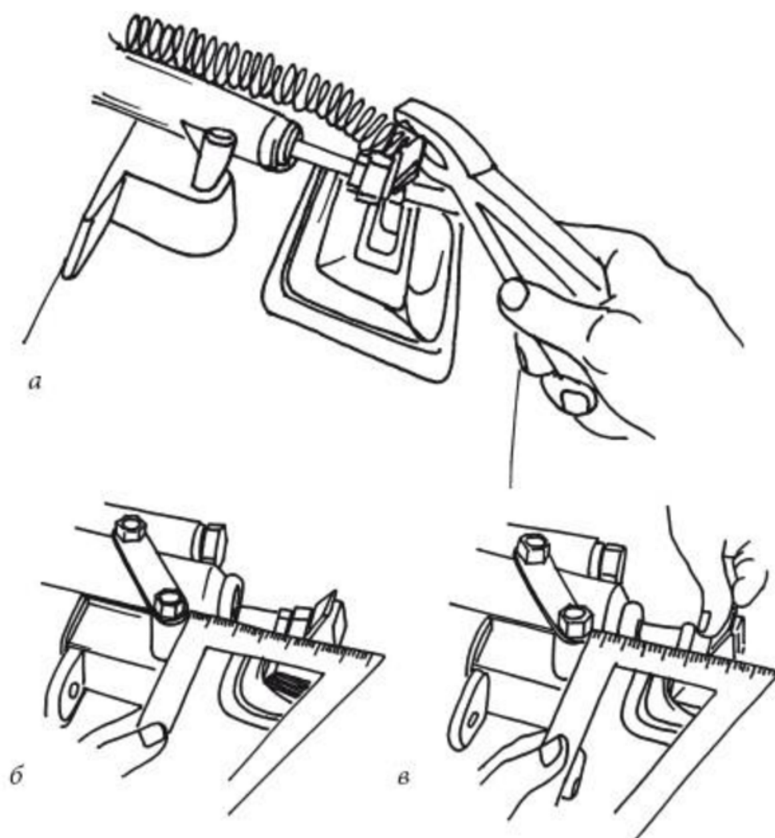
Рисунок 8. Проверка свободного хода толкателя
