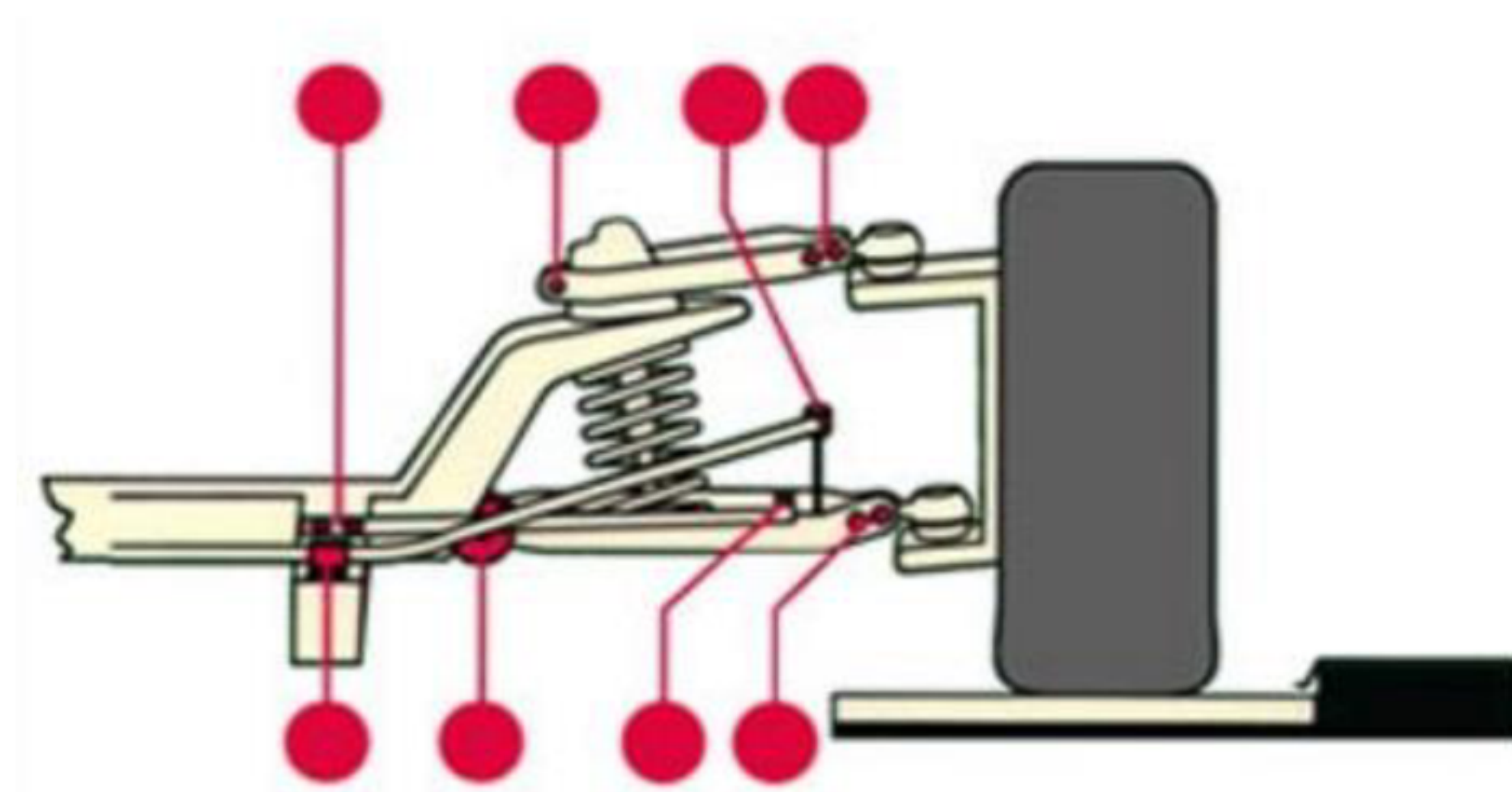
Рисунок 10. Точки контроля в подвеске автомобиля
