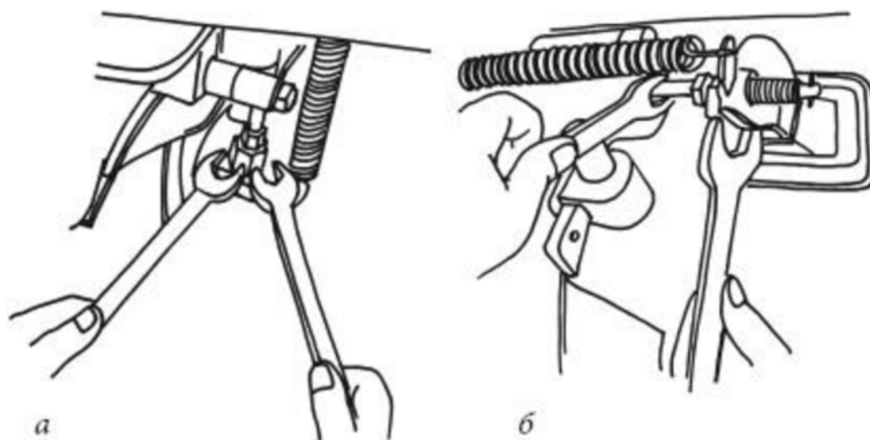
Рисунок 9. Регулировка свободного хода толкателя
