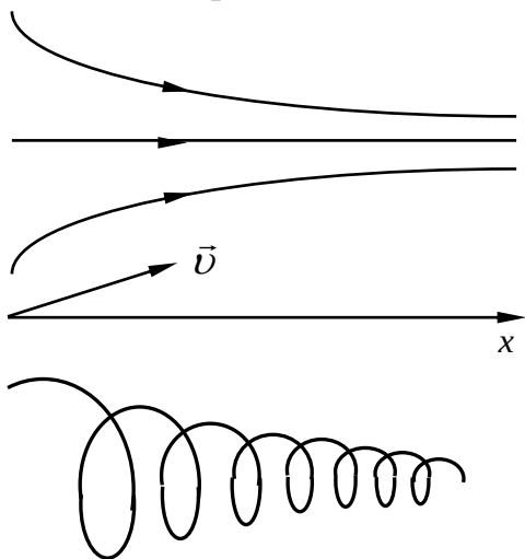
Рис.5. Движение заряженной частицы в неоднородном магнитном поле
