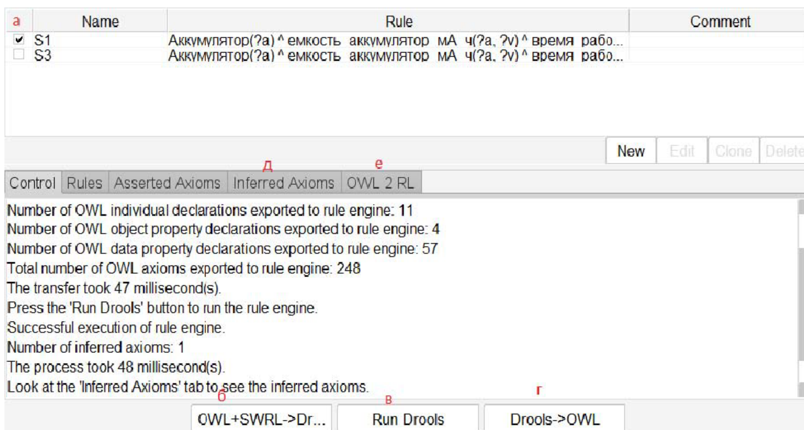
Рис. 26 Вкладка SWRL в системе Protégé (а – активность правила; б – кнопка загрузки понятий/аксиом из онтологии и списка правил; в – запуск вывода на основе правил; г – внесение выведенных понятий в онтологию; д – список
