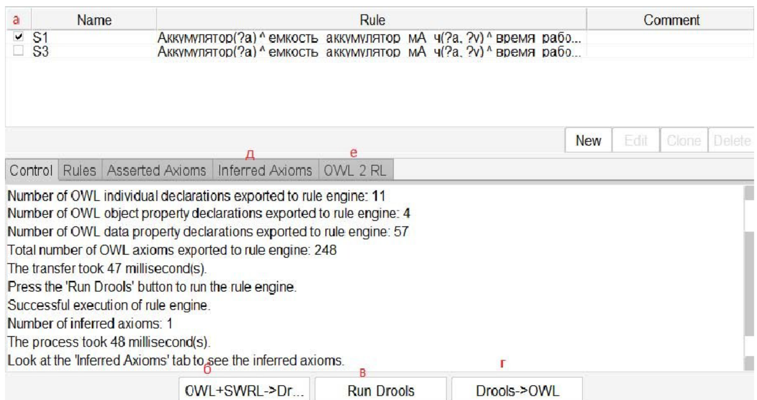
Рис. 26 Вкладка SWRL в системе Protégé (а – активность правила; б – кнопка загрузки правил; в – запуск вывода на основе правил; г – внесение выведенных понятий в онтологию; д – список правил)
