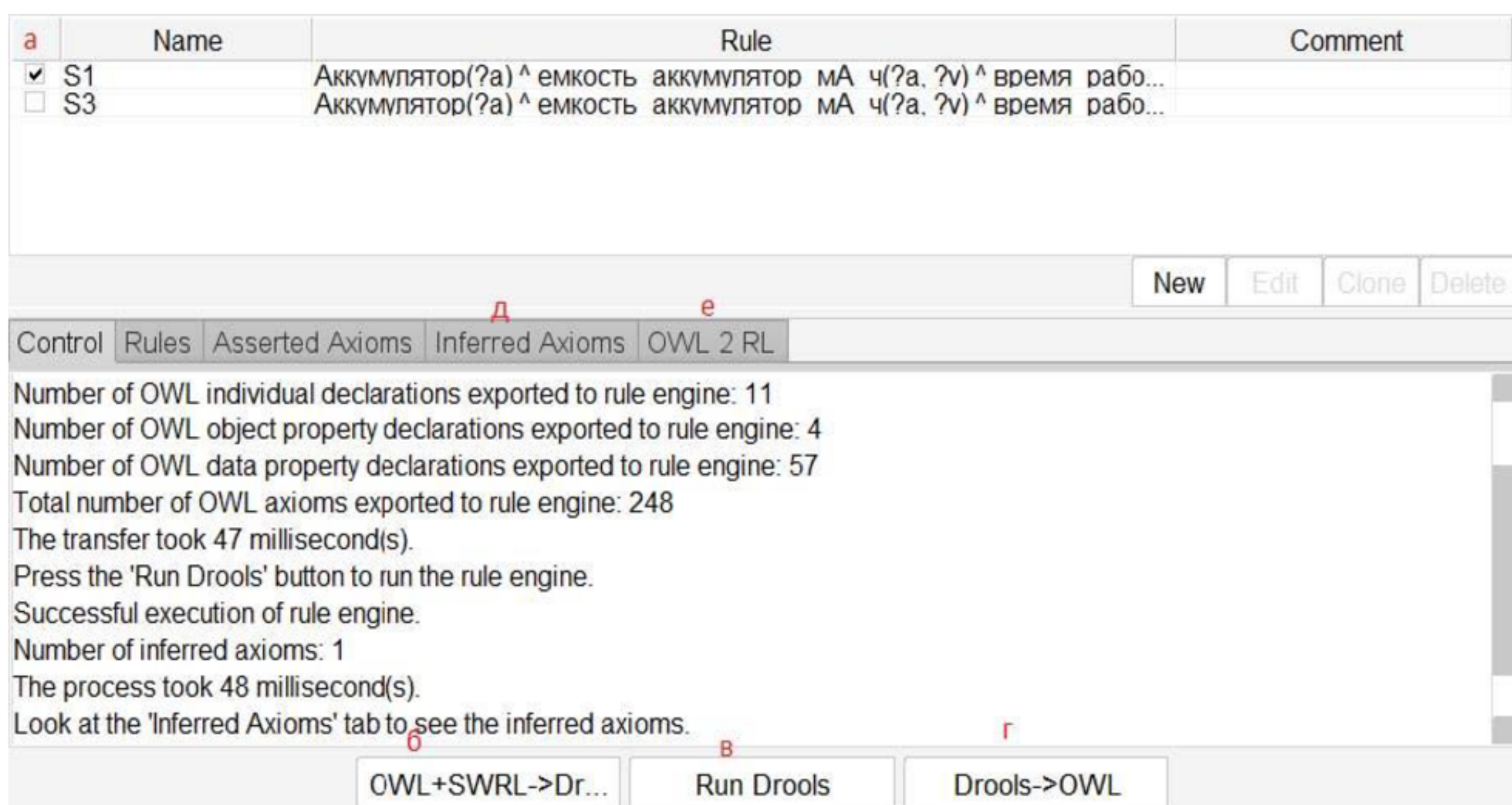
Рис. 26 Вкладка SWRL в системе Protégé (а – активность правила; б – кнопка запуска правила; в – загрузка онтологии и списка правил; г – запуск вывода на основе правил; д – внесение выведенных понятий в онтологию; е – список
