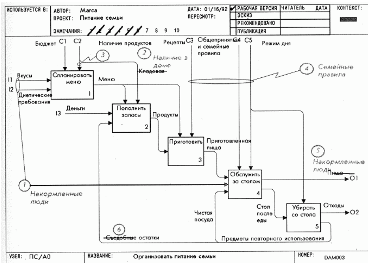
Рис. 7. Критическая оценка диаграммы А0
