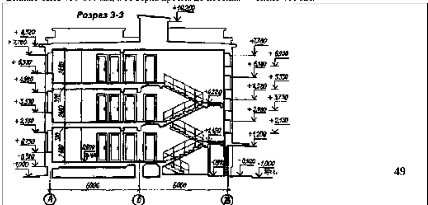
Рисунок 10.1 Архитектурный разрез
