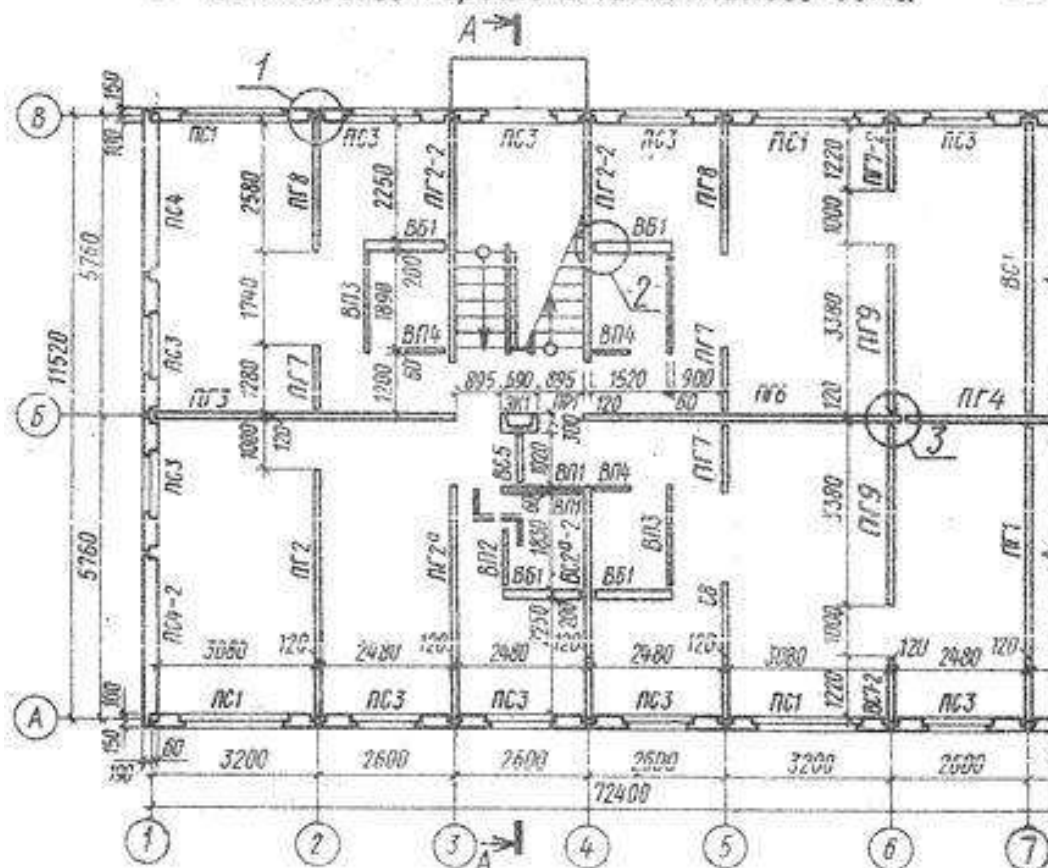
Схема расположения панелей стен, перегородок, вентблоков первого этажа жилого дома
