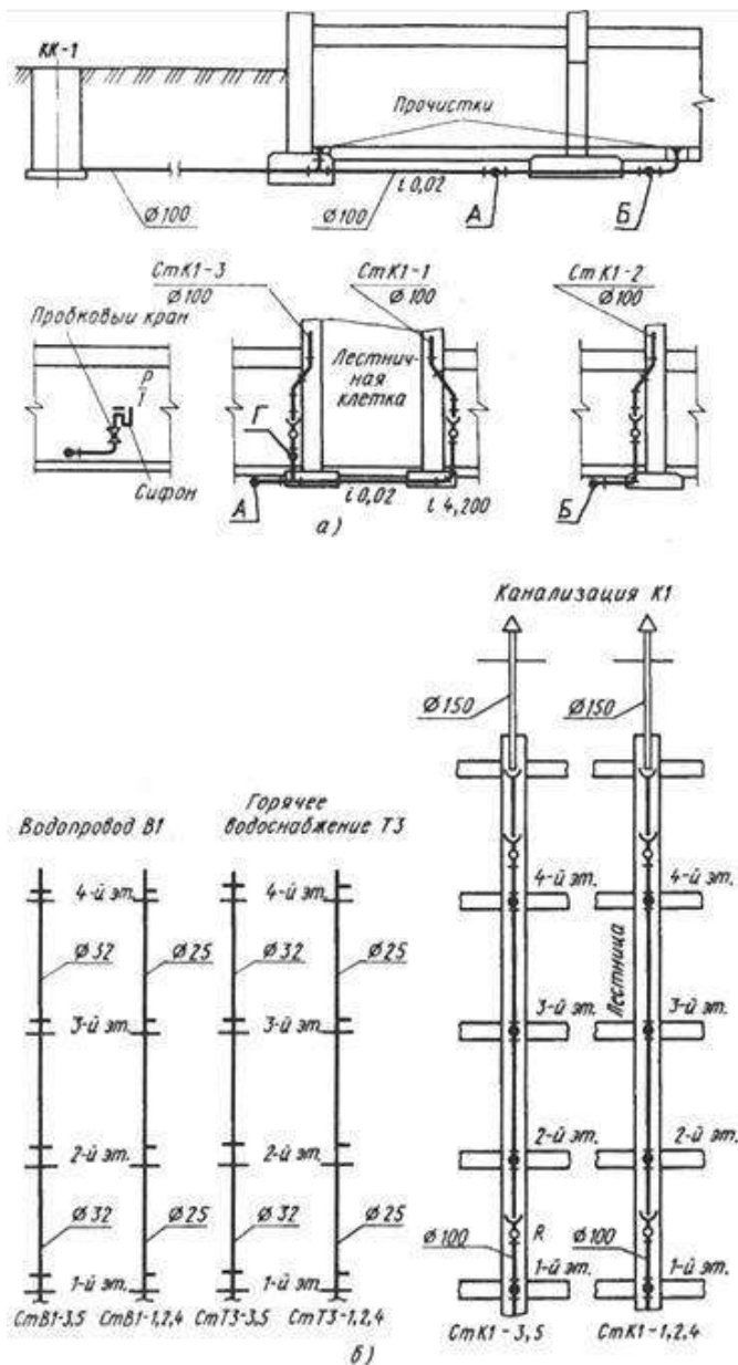
Рис. 18.5 Фрагмент монтажного плана санитарного узла.
