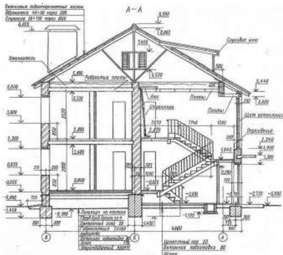
Разрез
