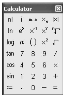
Рис2. Палитра вычислений.
