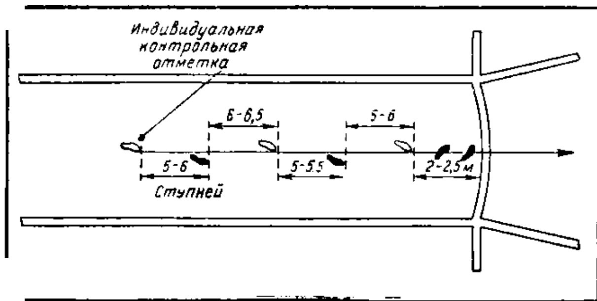
Рис.72. Линия для постановки ног
