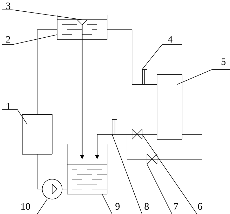
Схема установки
