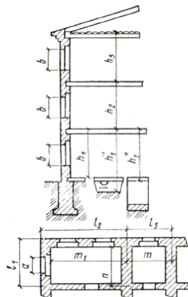
Рис. 1. Смеха обмера теплопередающих ограждений
