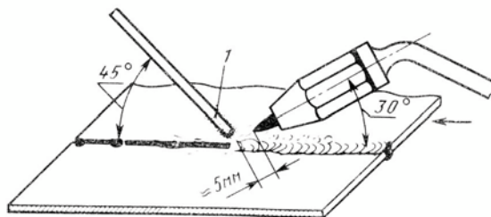
Рис. 5. Расположение горелки и припоя при пайке латунным припоем: Л – порошковый флюс, нанесенный на конец припоя или пруток, покрытый флюсом
