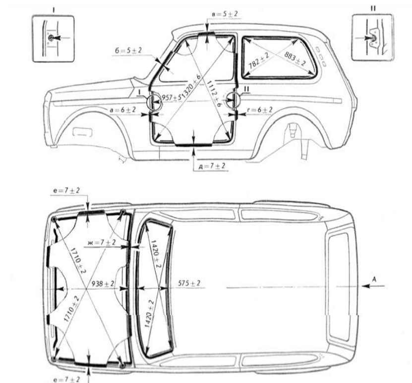
Рис. 7. Размеры проемов и зазоры сопрягаемых деталей кузова автомобиля модели ВАЗ-2121
