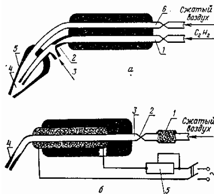
Рис. 2. Схема горелок для сварки термопластов горячими газами: а – газовая горелка ГПИ-1-56; б – газозлектрическая горелка
