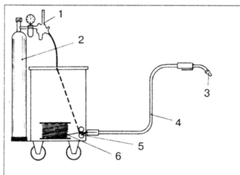
Рис. 10. Схема аппарата для сварки в среде защитного газа: 1 – редуктор; 2 – газовый баллон; 3 – горелка; 4 – направляющий шланг; 5 – электрод; 6 – деталь
