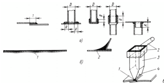
Рис. 3. Пайка оловянным припоем:
