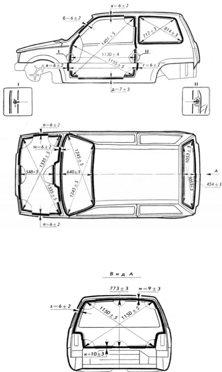
Рис. 9. Размеры проемов и зазоры спрягаемых деталей кузова автомобиля модели ВАЗ-1111
