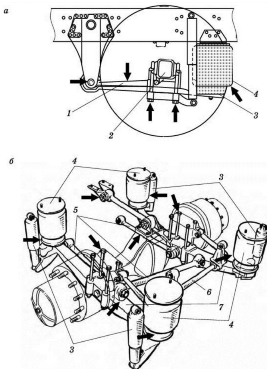
Рисунок 5. Варианты исполнения пневмоподвесок неуправляемых осей и основные места их контроля:
