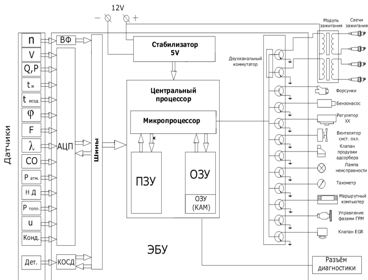
Рис 1. Блок-схема управления впрыском топлива и зажигания: n – датчик частоты вращения и положения коленчатого вала; v – датчик скорости движения автомобиля; Q, P – датчик нагрузки на двигатель; t_{\text{ж}} – датчик температуры охлаждающей жидкости; t_{\text{возд.}} – датчик температуры воздуха; U – сигнал напряжения аккумуляторной батареи; \phi – датчик положения дроссельной заслонки; F – датчик фаз; \lambda – датчик кислорода; CO – потенциометр (может устанавливаться на автомобилях, на которых не установлен кислородный датчик); P_{\text{атм.}} – датчик атмосферного давления; Н Д – датчик неровности дороги; P_{\text{топл.}} – датчик давления топлива; U – сигнал напряжения бортовой сети; Конд. – сигнал включения кондиционера; Дет – датчик детонации.
