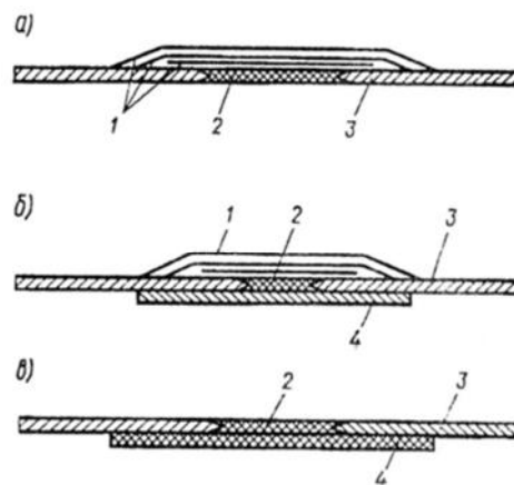
Рис. 1. Варианты устранения сквозных повреждений в панелях кузова путем установки накладок из стеклоткани:
