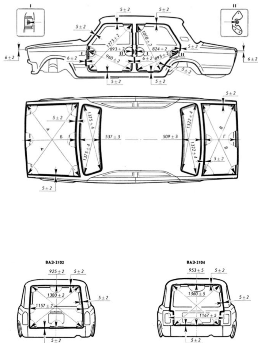
Рис. 6. Размеры проемов и зазоры сопрягаемых деталей кузова автомобилей моделей BA3-2101 - 2107
