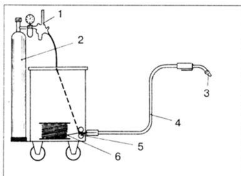
Рис. 10. Схема аппарата для сварки в среде защитного газа: 1 – редуктор; 2 – газовый баллон; 3 – горелка; 4 – направляющий шланг; 5 – электрод
