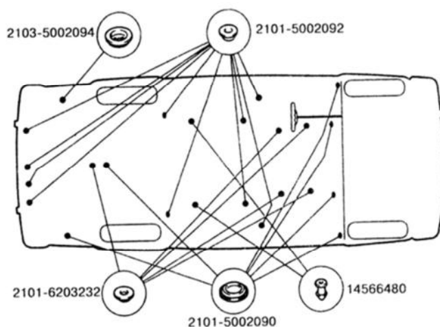
Рис. 22. Схема установки заглушек на кузове ВАЗ-2106
