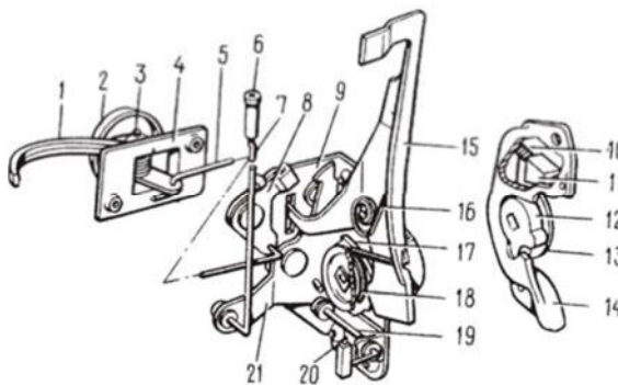
Рис. 1. Замок передней левой двери:
