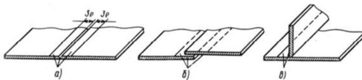
Рис. 4. Подготовка кромок к пайке латунным припоем: а – участки, зачищенные до металла; б и в – зачистка до чистого металла
