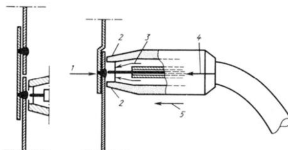
Рис. 11. Положение горелки при сварке в среде защитного газа
