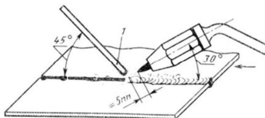
Рис. 5. Расположение горелки и припоя при пайке латунным припоем: I – порошковый флюс, нанесенный на конец припоя или пруток, покрытый флюсом
