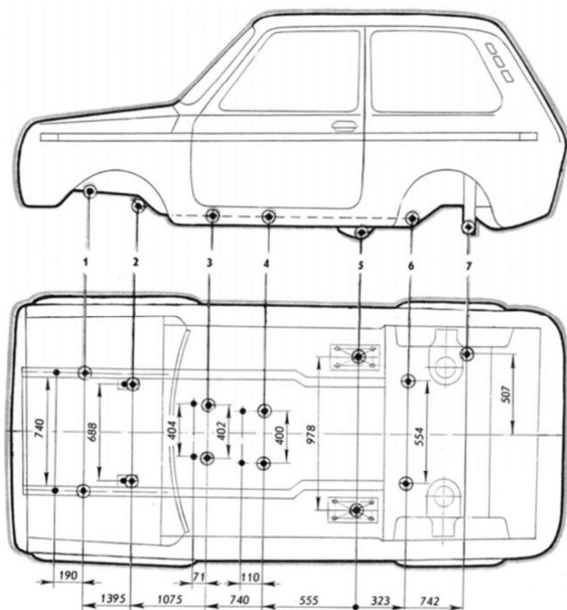
Рис. 11. Точки крепления двигателя и подвесок на кузове автомобиля модели ВА3-2121
