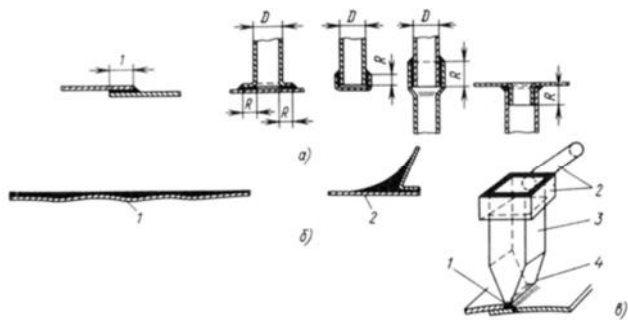
Рис. 3. Пайка оловянным припоем:
