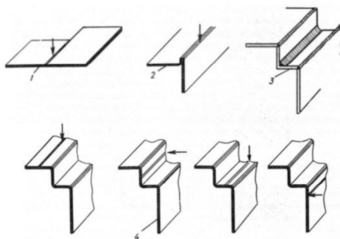
Рис. 6. Подготовка кромок тонких листов под сварку:
