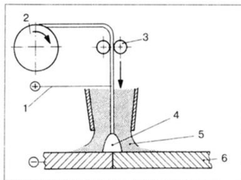
Рис. 9. Схема процесса сварки в среде защитного газа: 1 – электрод; 2 – катушка с проволочным электродом; 3 – механизм подачи проволочного электрода; 4 – электрическая дуга; 5 – защитный газ; 6 – деталь
