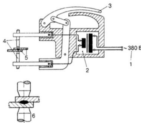
Рис. 13. Принципиальное схематическое изображение клещей для контактно-точечной сварки и сварной точки:
