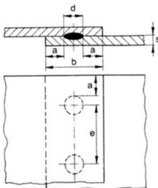
Рис. 14. Геометрические параметры контактно-точечной сварки:
