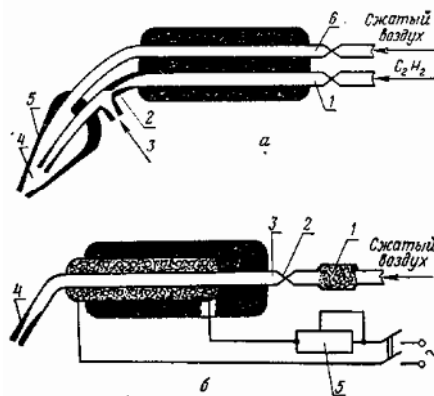
Рис. 2. Схема горелок для сварки термопластов горячими газами: а – газовая горелка ГПП-1-56; б – газозлектрическая горелка
