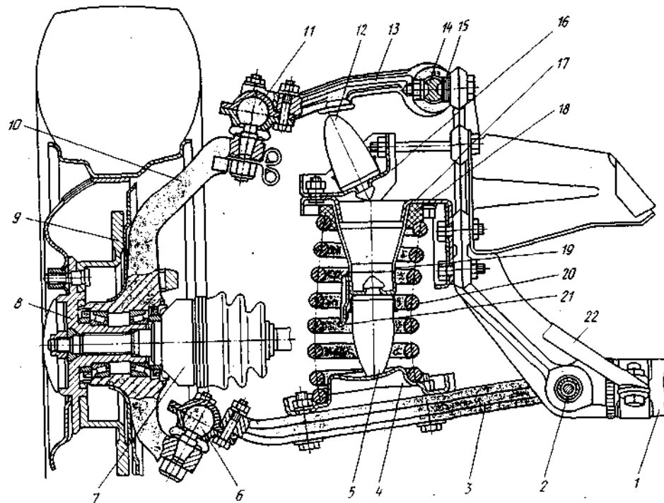
Рис. 22. Передняя подвеска легкового автомобиля ВАЗ-2121 «Нива»: 1 — поперечина; 2 — ось нижнего рычага; 3 — нижний рычаг; 4 и 17 — соответственно нижняя и верхняя опорные чашки пружины; 5 — буфер сжатия; 6 и 11 — соответственно нижний и верхний шаровые шарниры; 7 — наружный шарнир привода переднего колеса; 8 — ступица; 9 — тормозной диск; 10 — поворотный кулак; 12 — буфер отдачи; 13 — верхний рычаг; 14 — ось верхнего рычага; 15 — регулировочные прокладки; 16 — кронштейн; 18 — виброшумоизолирующая прокладка; 19 — опора; 20 — пружина; 21 — упор; 22 — растяжка
