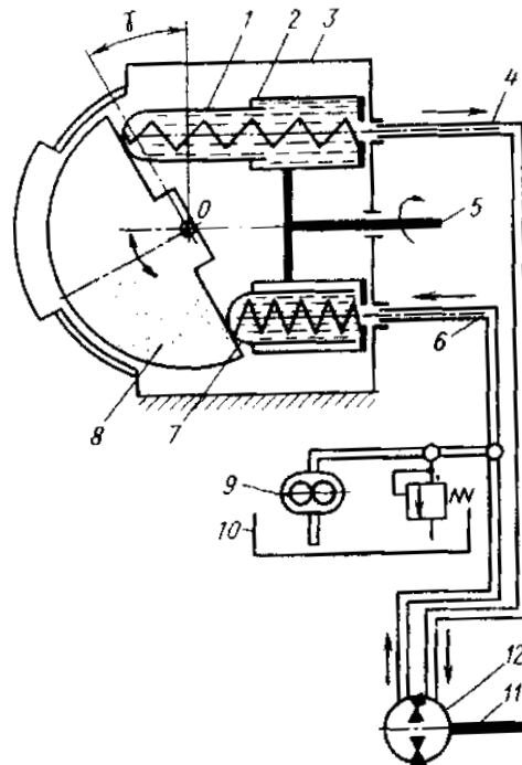
Рис. 6. Схема гидрообъемной коробки передач
