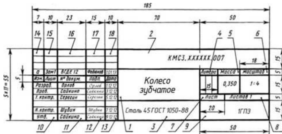
Рисунок 1 Основная надпись чертежа
