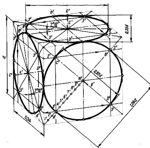
Рисунок 10 Окружность в диметрии
