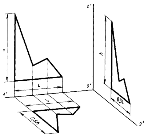
Рисунок 9 Фигура в диметрии
