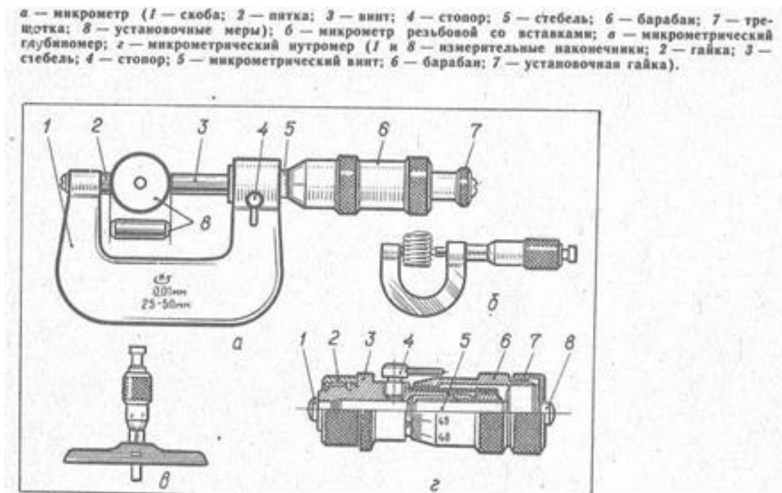
Рис. 14.3 Микрометрические инструменты
