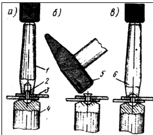
Рис.10.4. Рабочие операции клепки: а - осаживание соединяемых листов; б - расклепка стержня заклепки молотком; в - формирование головки; 1 - осадка; 2 - заклепка; 3 - заклепываемые листы; 4 - поддержка; 5 - молоток; 6 - обжимка
