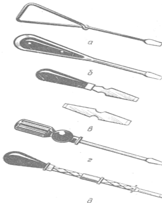
Рис. 18.2. Отвертки: а-проволочная; б — с деревянными щечками; в- вставная; г- электротехническая; д — механическая
