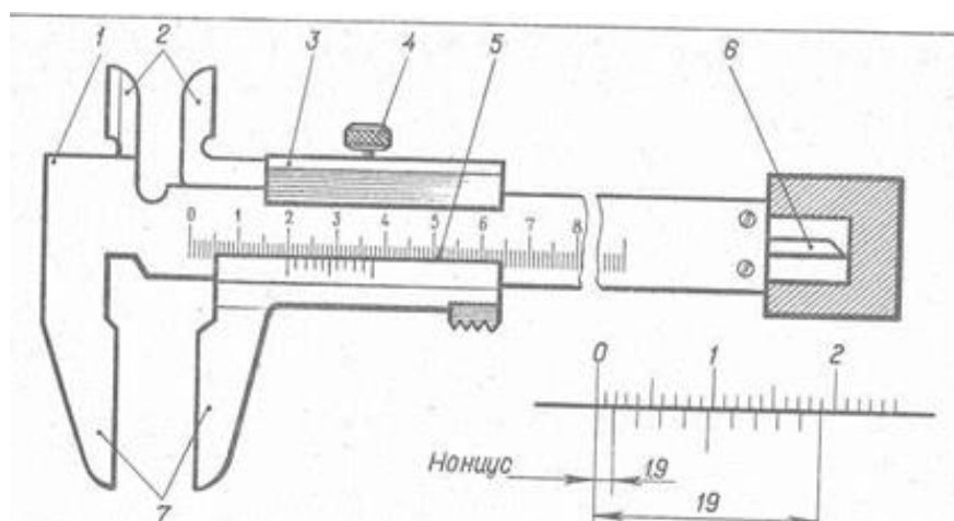
Рис. 14.1 Штангенциркуль ШЦ-1:
